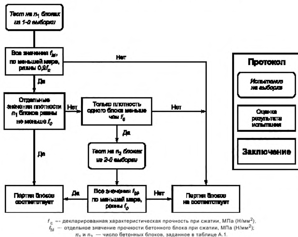
Рисунок В.3 — Схема для оценки характеристической прочности блоков
