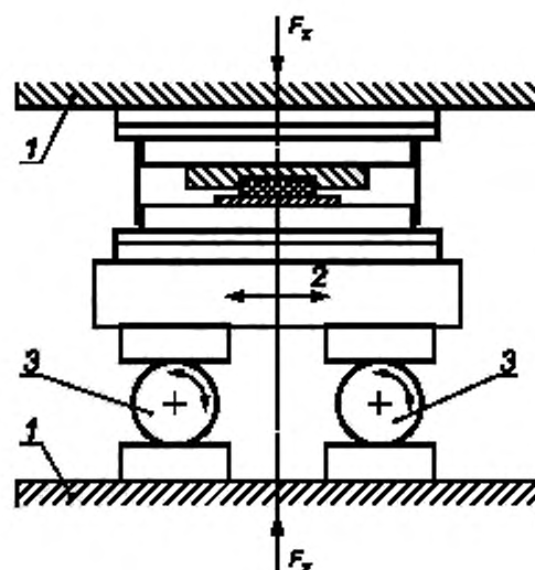
1 — пластины испытательного пресса; 2 — подвижная пластина, 3 — роликовые подшипники
