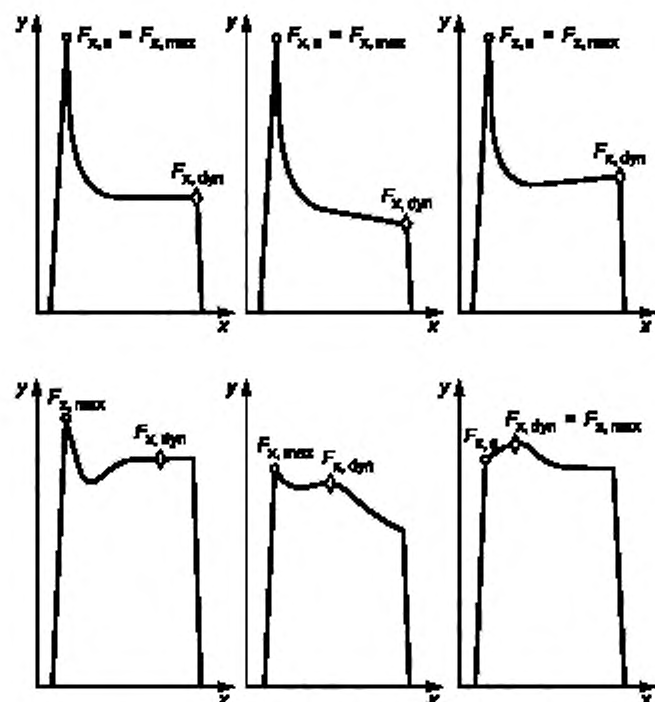
а) Скользящие части со смазанным ПТФЭ по аустенитной стали или стали с твердым хромированием
