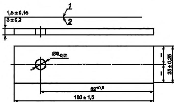
1 — наружные стыкующиеся детали; 2 — внутренняя стыкующаяся деталь
