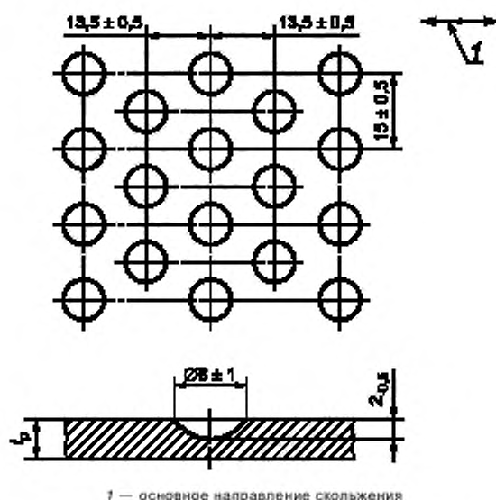
Рисунок 1 — Карманы для смазки в разделенных на камеры плитах из ПТФЭ
