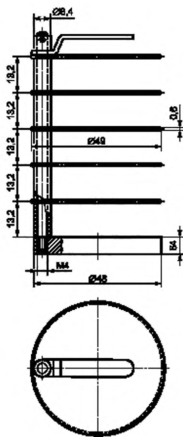
Рисунок Н.3 — Держатель для чашки
