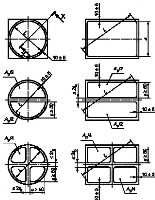
Рисунок 3 — Примеры изображения ячеистых ровных плит из ПТФЭ
