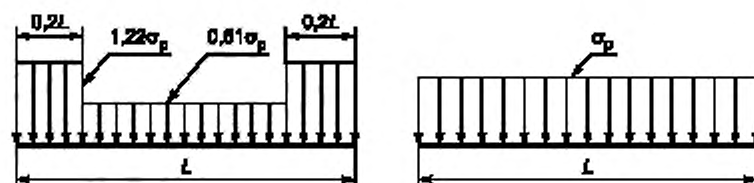
Рисунок 10 — Альтернативное распределение нагрузки при сжатии ПТФЭ
