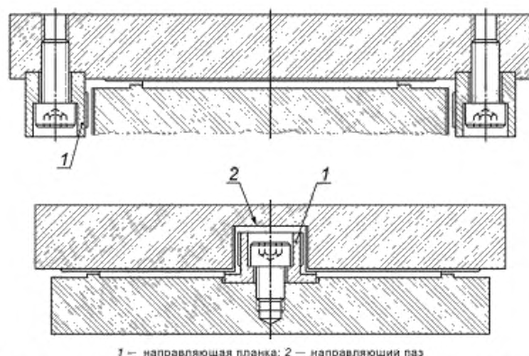
1 — направляющая планка; 2 — направляющий паз Рисунок 7 — Типовые примеры расположения свинчивающихся направляющих
