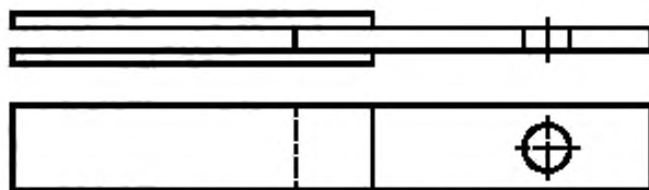
Рисунок 1.1 — Склейка наложением с двумя срезами
