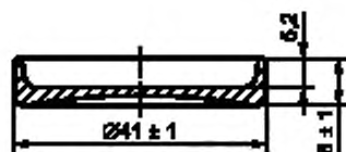
Рисунок Н.2 — Чашка
