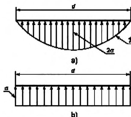
Рисунок 11 — Распределение нагрузки при сжатии эластомера
