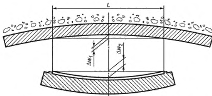
Рисунок 9 — Относительные деформации несущих пластин
