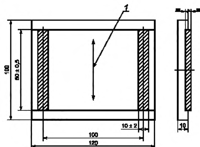
Рисунок D.3 — Испытательный образец многослойных материалов
