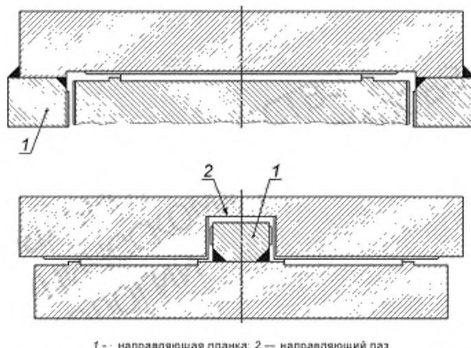
Рисунок 8 — Типовые примеры расположения сварных направляющих
