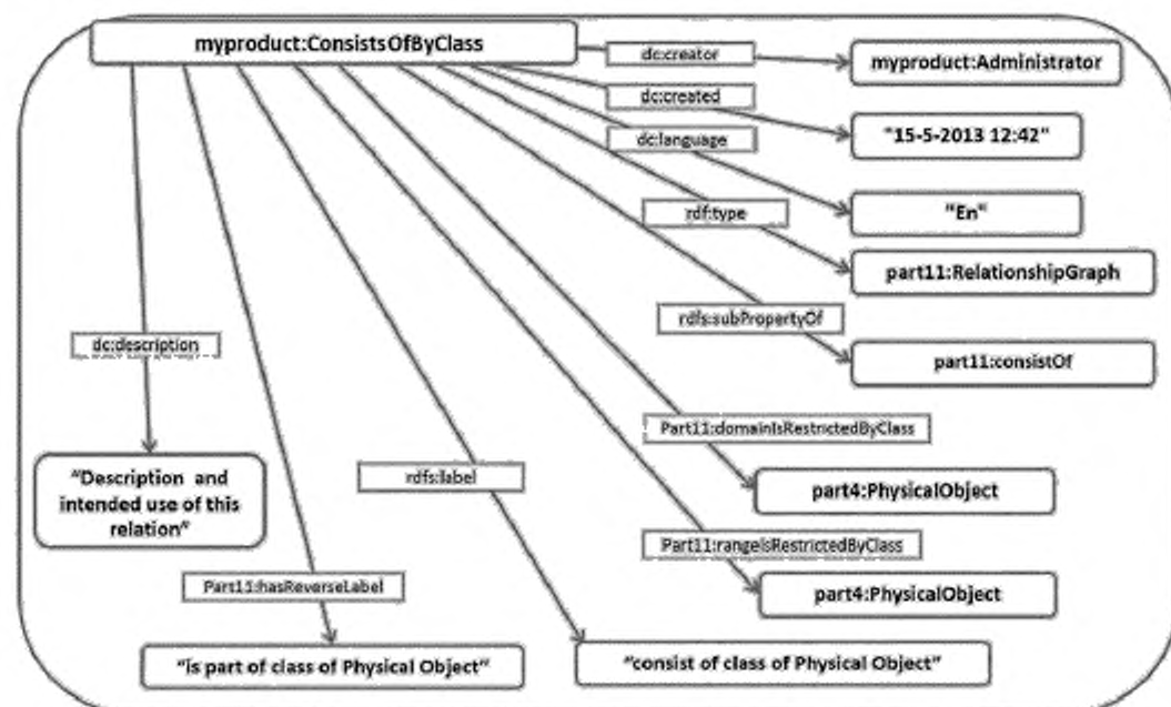
Рисунок 44 — Именованный RDF-граф, специализирующий взаимосвязь part11:consistsOf для взаимосвязи myproduct:ConsistsOfByClassOfPhysicalObject
