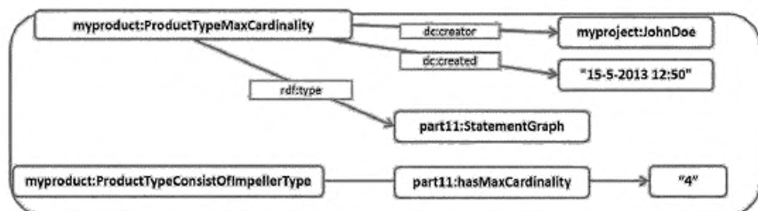
Рисунок 51 — Именованный RDF-граф, указывающий на то, что экземпляр класса myproduct:PumpType состоит как максимум из четырех экземпляров myproduct:ImpellerType «4»
