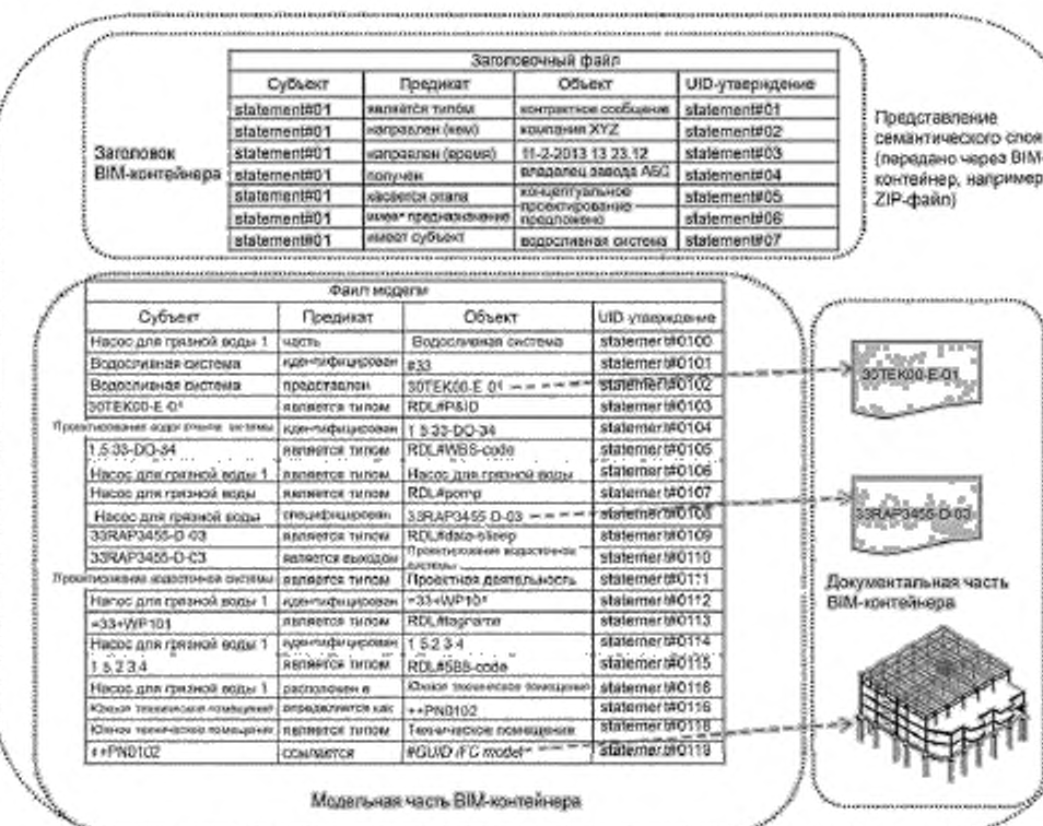
Рисунок С.2 — Пример структуры и содержания BIM-контейнера на основе настоящего стандарта
