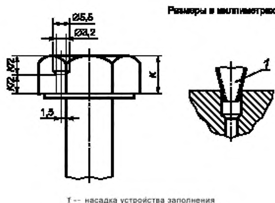
Рисунок J.2 — Отверстие в головке болта
