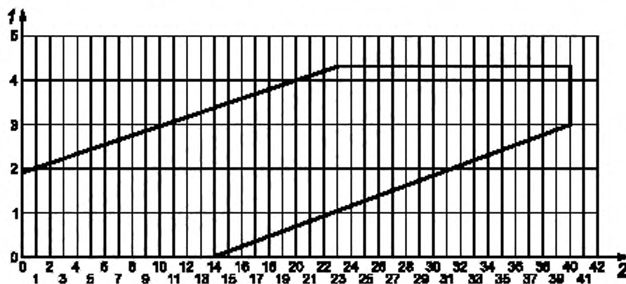
Рисунок L.3 — Схема последовательного контроля типа Б
