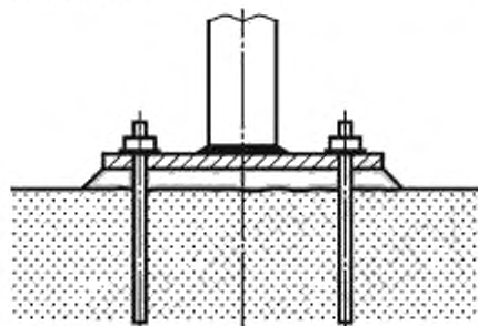
Рисунок 6 — Цементирование под опорной плитой
