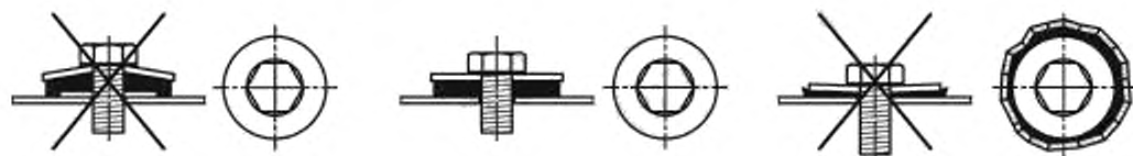
Рисунок 5 — Рекомендации по установке уплотнительных шайб
