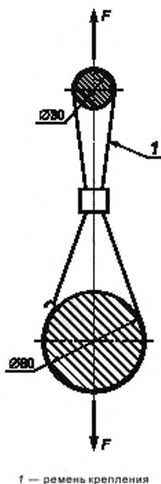
Рисунок А.1 — Комплект для испытаний ремней крепления
