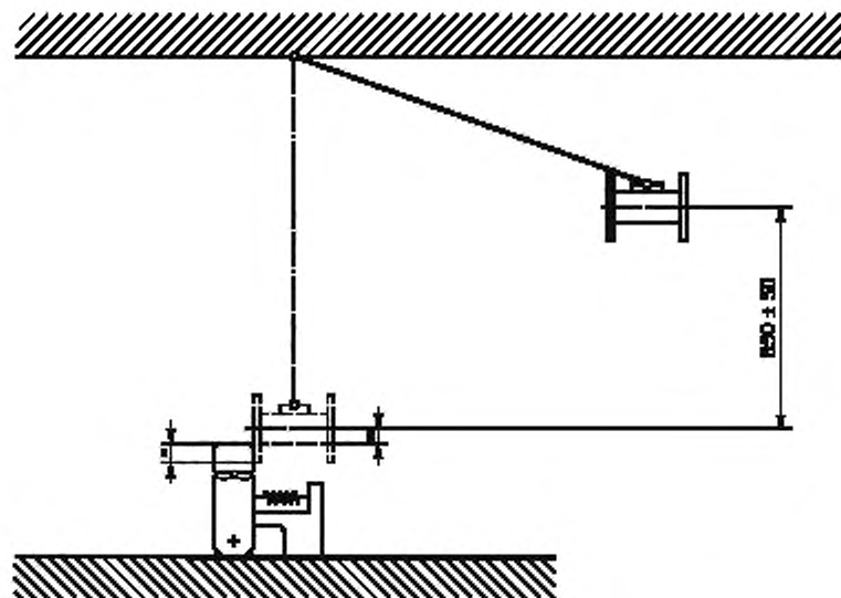
Рисунок 5 — Испытание прочности тормозного устройства
