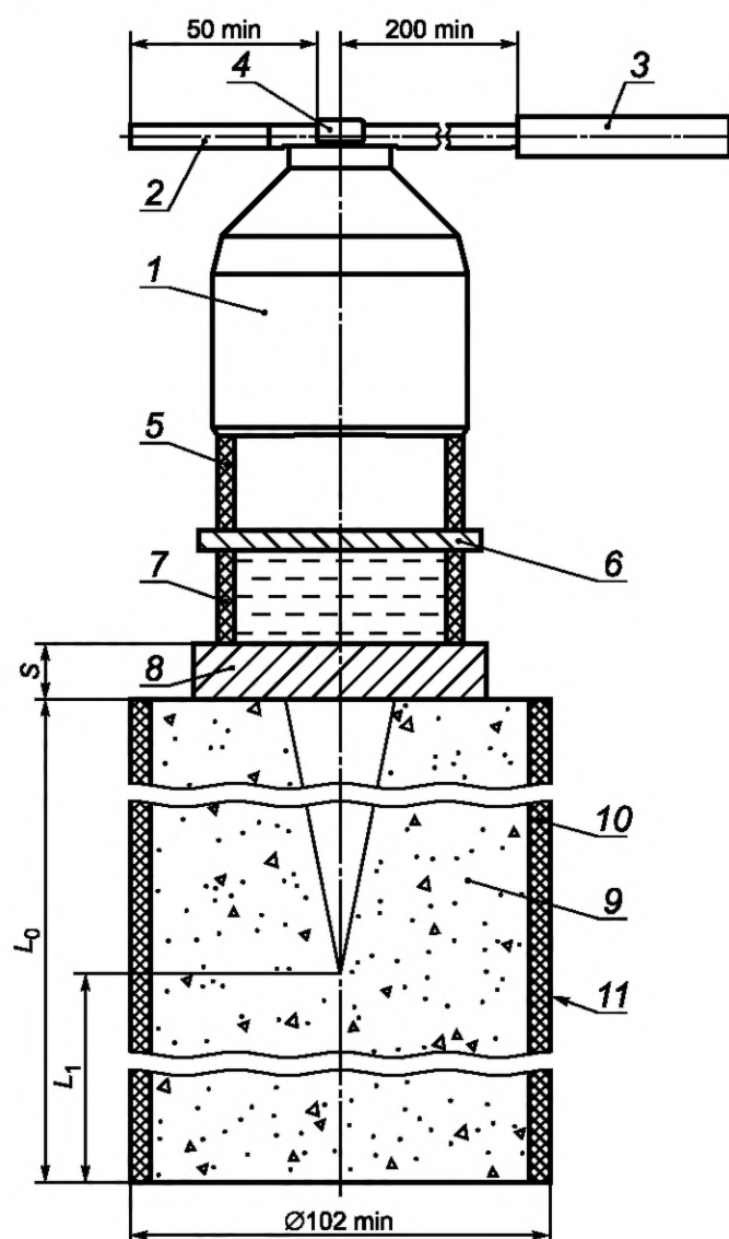
1 — КЗ; 2 — отрезок ДШ; 3 — средство инициирования; 4 — фиксатор или липкая лента; 5 — втулка-фокус; 6 — стальная пластина Б, имитирующая корпус перфоратора; 7 — втулка-клиренс с водой; 8 — стальная пластина А, имитирующая обсадную колонну; 9 — бетонная мишень МККБ; 10 — гильза; 11 — полиэтиленовый рукав
