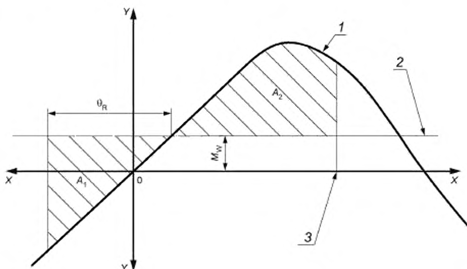
X — угол крена, °; Y — восстанавливающий или кренящий момент, кН·м; 1 — восстанавливающий момент, кН·м; 2 — кренящий момент, вызванный ветровой нагрузкой, кН·м; 3 — \theta_{A2} = \theta_{DA} или 50^\circ , что меньше, или второй установившийся угол крена, вызванный ветровой нагрузкой
