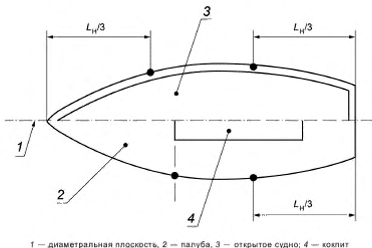
Рисунок F.1 — Расположение испытательных грузов
