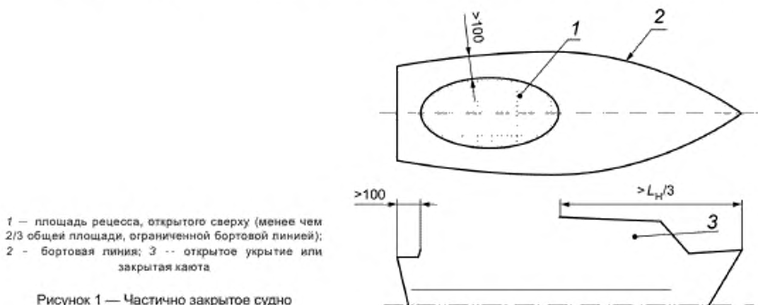
Рисунок 1 — Частично закрытое судно
