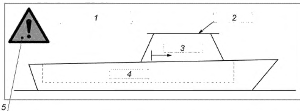
1 — текст, устанавливающий максимальное число людей на борту; 2 — текст, устанавливающий ограничения доступа, такие, как «Сидеть или стоять запрещено»; 3 — текст, устанавливающий ограничения доступа, такие, как «Максимальное количество людей на палубе — 2»; 4 — текст, устанавливающий ограничения доступа, такие, как «Нет ограничений»; 5 — знак W001 «Общее предупреждение» из ISO 7010
