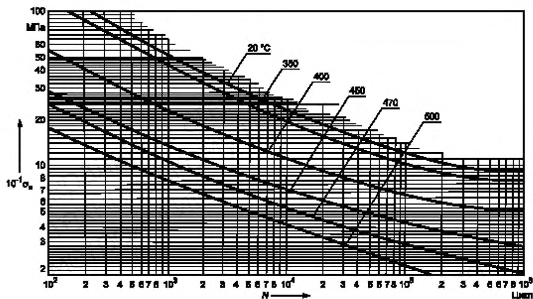
Рисунок 2 — Расчетные кривые малоциклового усталости углеродистых сталей
