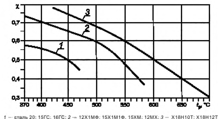
Рисунок 5 — Коэффициент усреднения компенсационных напряжений
