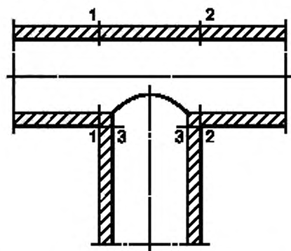
Рисунок 12 — Расчетные сечения тройникового узла
