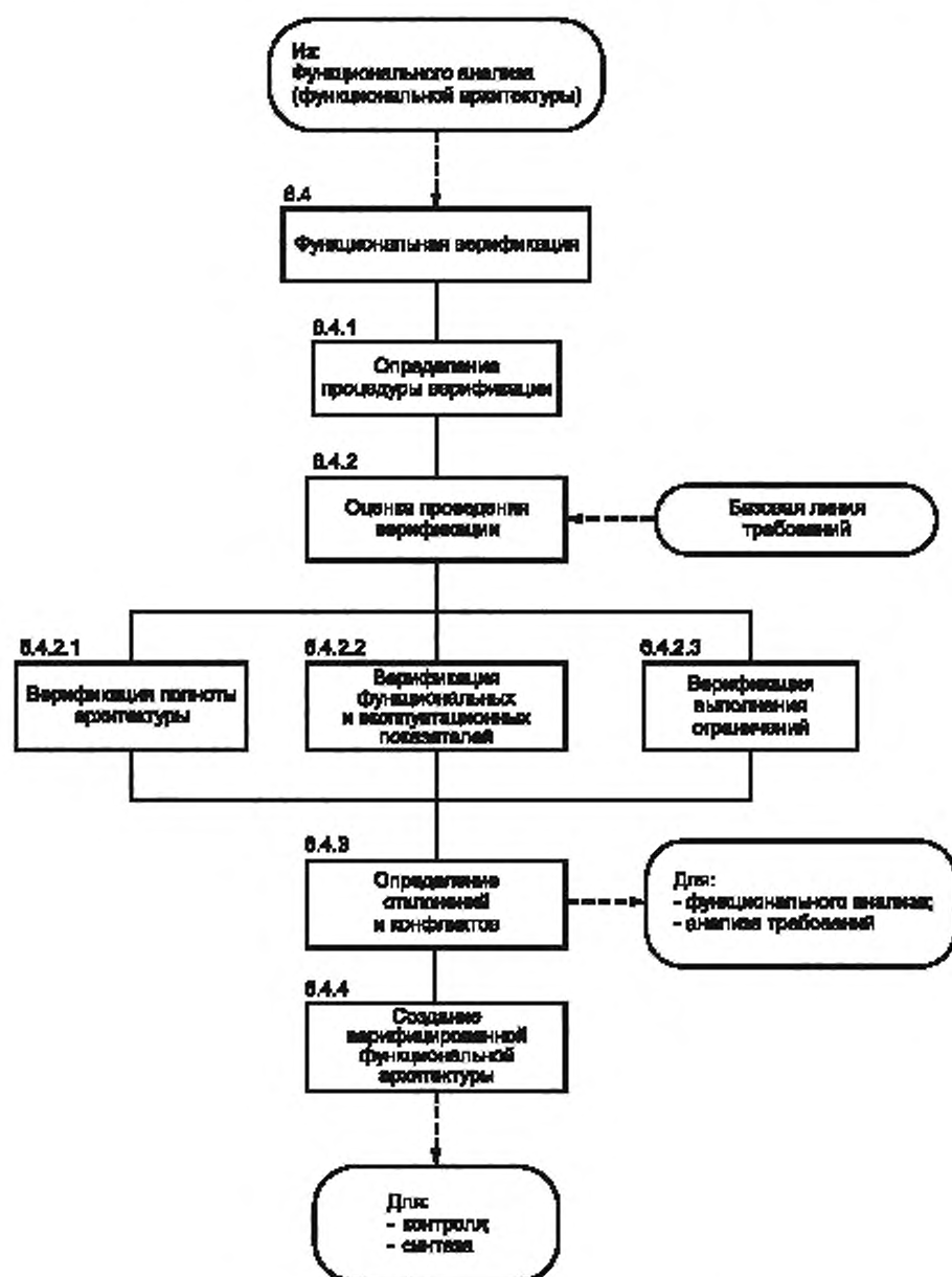
Рисунок 13 — Функциональная верификация
