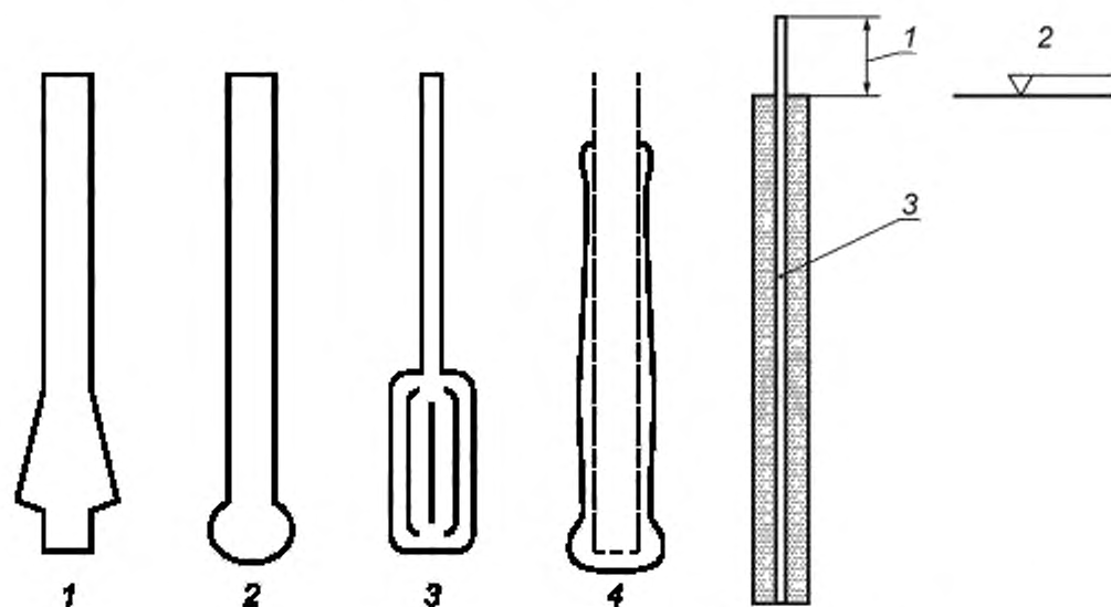
1, 2 — буровая микросвая с уширенной пяткой; 3 — микросвая с уширенным стволом; 4 — микросвая с расширением путем цементирования
