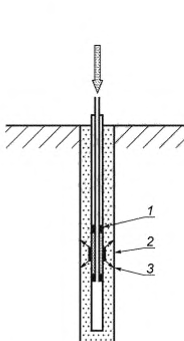
1 — пакер; 2 — клапаны для инъекции 3 — направления распространения раствора
