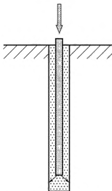
Рисунок 6c) — Одноэтапное нагнетание через несущий элемент
