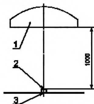
1 — ИЗДЕЛИЕ; 2 — ЦЕНТР СВЕТОВОГО ПОЛЯ (ЦСП); 3 — головка фотометра
