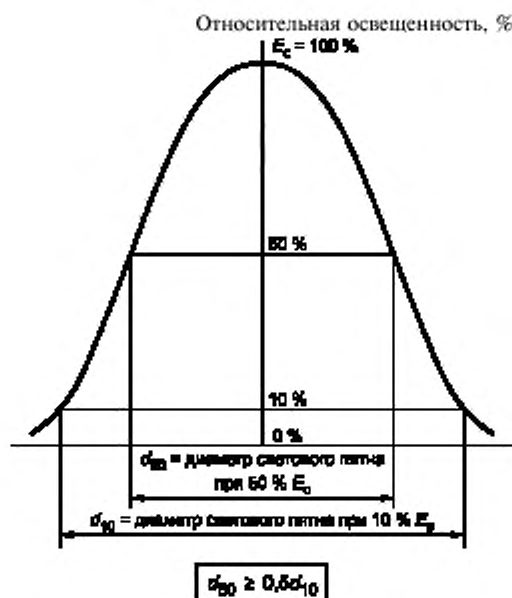
Рисунок 104 — Распределение света
