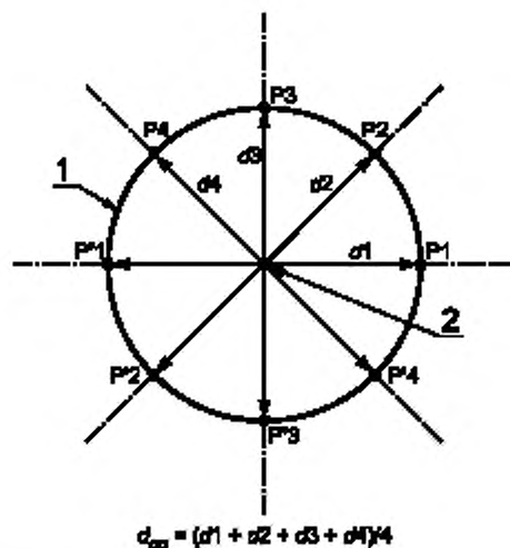
1 — диаметры, для освещенности достигает 10 % или 50 % ЦЕНТРАЛЬНОЙ ОСВЕЩЕННОСТИ; 2 — точка измерения, ЦЕНТР СВЕТОВОГО ПОЛЯ (ЦСП); P1 (P'1) — поперечное сечение 1; P2 (P'2) — поперечное сечение 2; P3 (P'3) — поперечное сечение 3; P4 (P'4) — поперечное сечение 4
