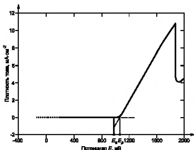
Рисунок 1 — Кривая зависимости плотности тока от потенциала, показывающая начало тока коррозии при E_a и потенциал пробы E_p
