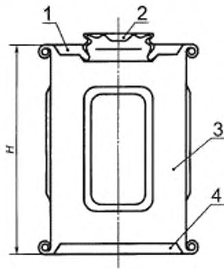
Рисунок 6 — Фляга типа II с опорными обручами
