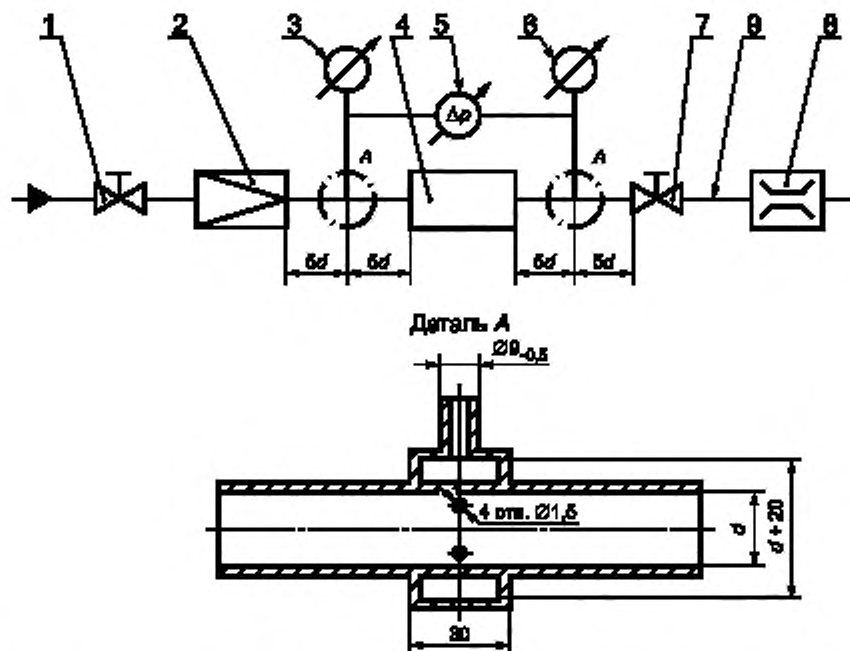
1, 7 — регулирующий клапан; 2 — регулятор входного давления; 3, 6 — манометры; 4 — испытуемое multifunctional регулирующее устройство; 5 — дифференциальный манометр; 8 — расходомер; 9 — точка измерения температуры
