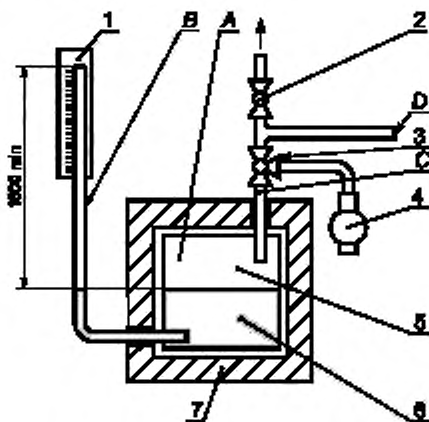
А — теплоизолированный сосуд давления; В — измерительная трубка; С — трубка под давлением; D — соединение с испытываемым клапаном; 1 — шкала; 2 — вентиль; 3 — трехходовой кран; 4 — компрессор; 5 — воздушная полость объемом 1 дм 3 ; 6 — вода; 7 — теплоизоляция
