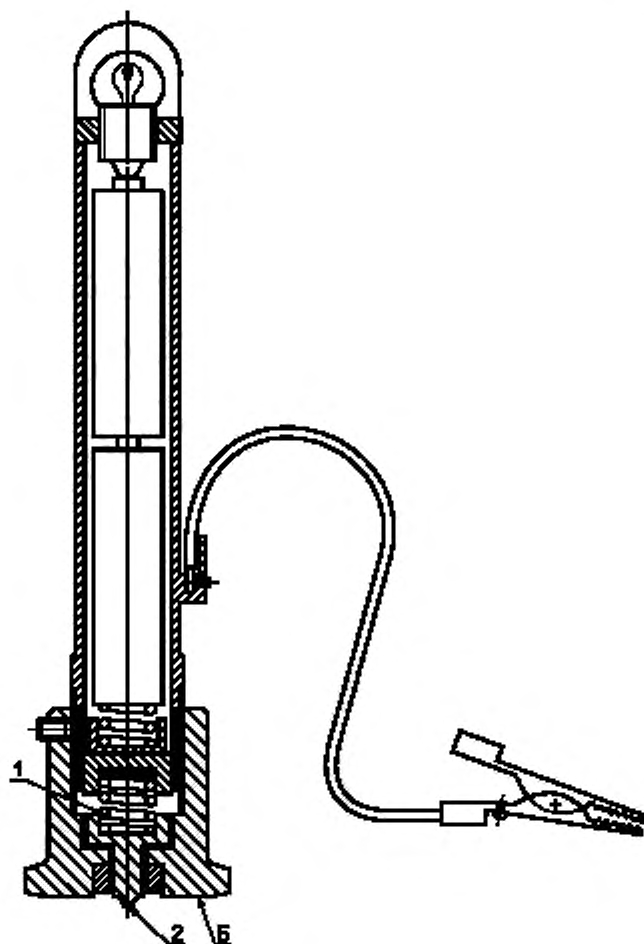
Б — поверхность испытываемого устройства; 1 — пружина с усилием нагрузки 10 Н; 2 — наконечник, которым проводится царапание (стальная сфера диаметром 1 мм);
