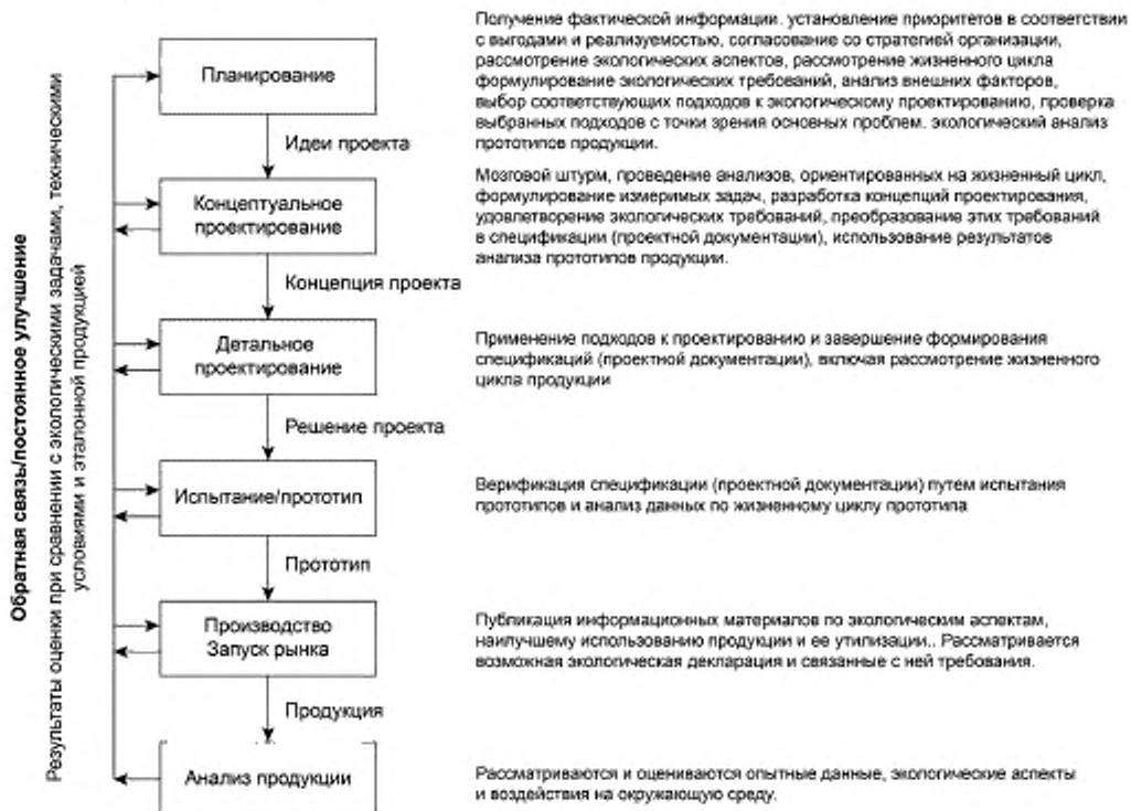
Рисунок 2 — Пример общей модели интегрирования экологических аспектов в процесс проектирования и разработки продукции
