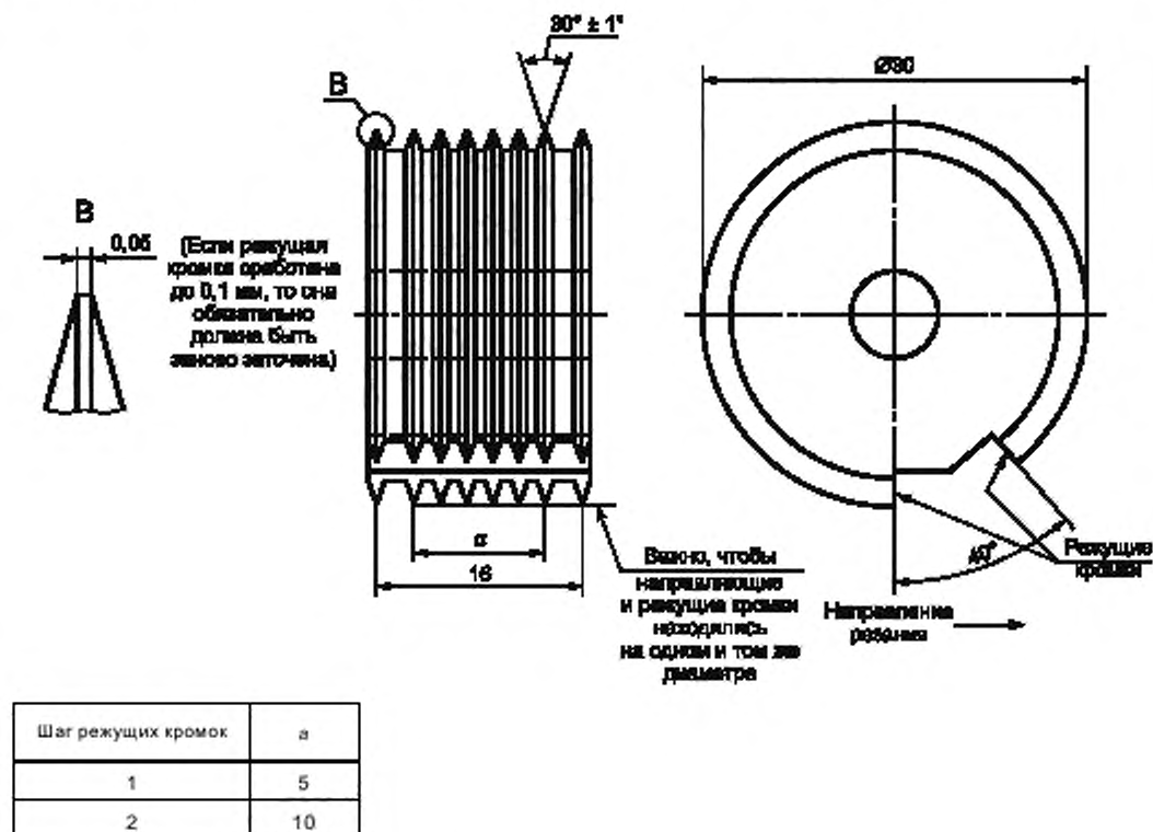
Рисунок 9 — Многолезвийный режущий инструмент
