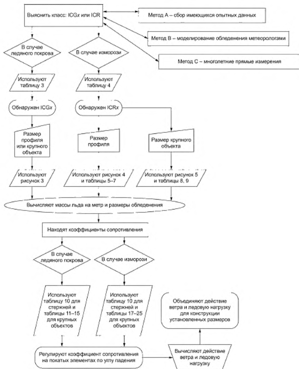
Рисунок Е.1 — Блок-схема процедуры расчета
