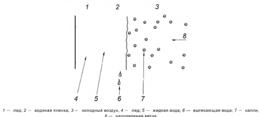
Рисунок С.3 — Образование гололеда («влажный прирост»)
