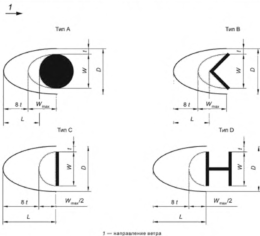
Рисунок 4 — Модель изморозевого обледенения (лист 1)
