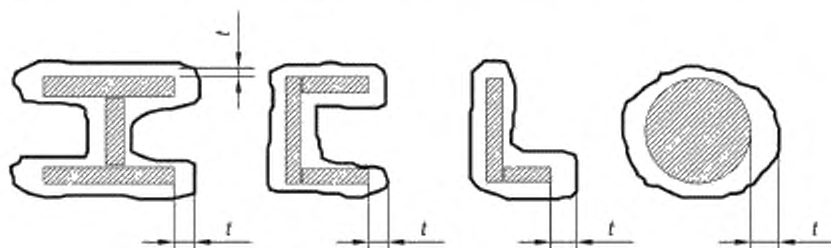
Рисунок 3 — Модель гололедного обледенения
