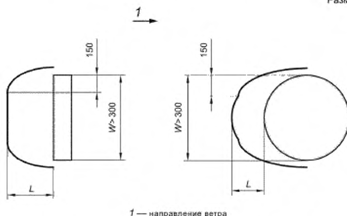
Рисунок 5 — Модель изморозевого обледенения для больших объектов
