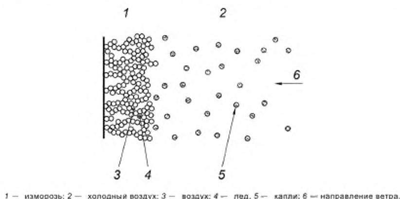
Рисунок С.2 — Образование изморози («сухой прирост»)
