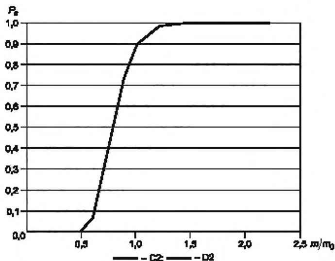
Рисунок D.8 — Оперативная характеристика P_a
