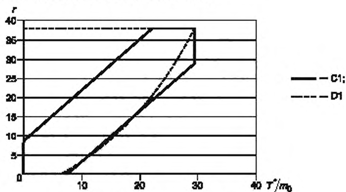
Рисунок D.1 — Линии приемки и отклонения
