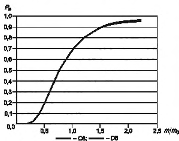
Рисунок D.32 — Оперативная характеристика P_a
