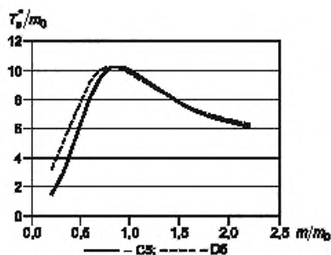
Рисунок D.18 — Зависимость T_e^*/m_0 от m/m_0
