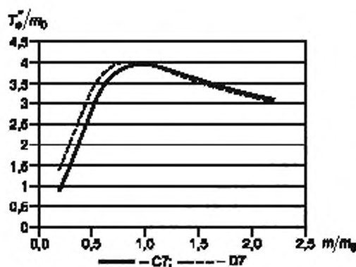
Рисунок D.26 — Зависимость T_e^*/m_0 от m/m_0
