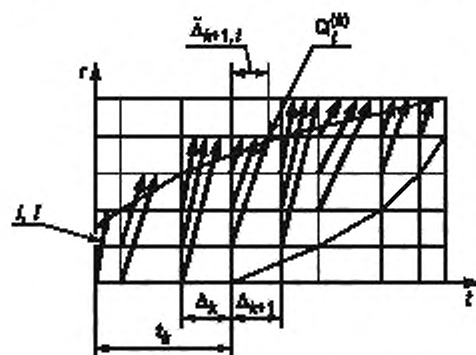
Рисунок К.6 — Путь до линии отклонения
