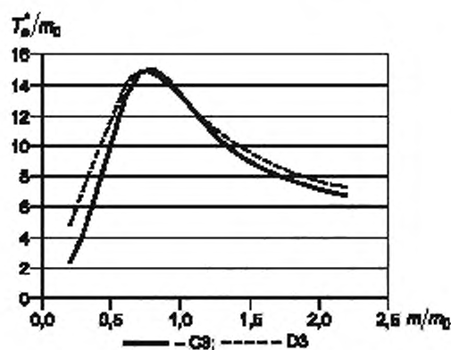
Рисунок D.10 — Зависимость T_e^*/m_0 от m/m_0
