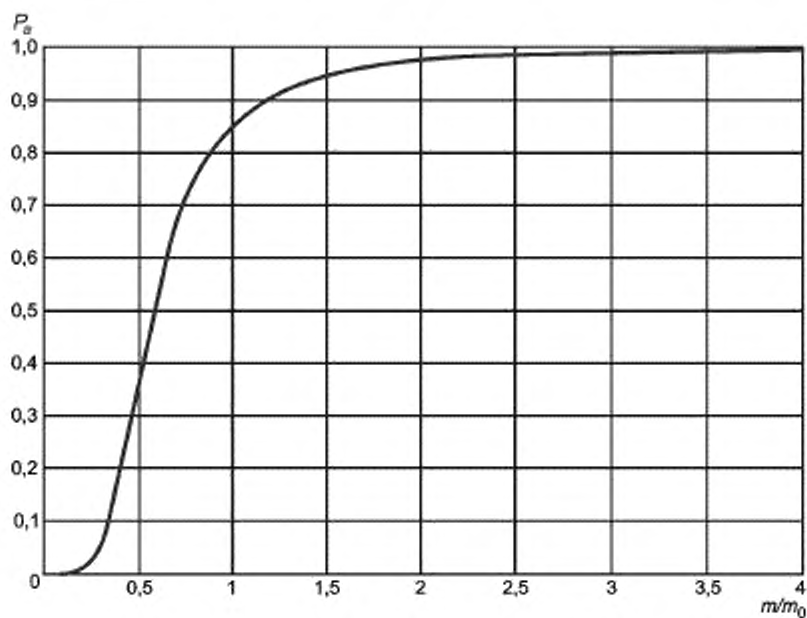
Рисунок A.8 — Кривая оперативной характеристики для плана испытаний A.3
