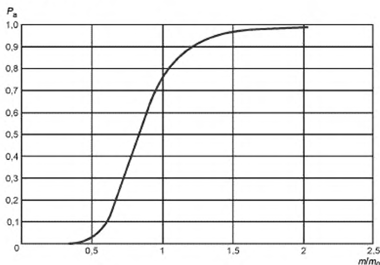
Рисунок F.2 — Кривая оперативной характеристики для вероятности приемы P_a .
