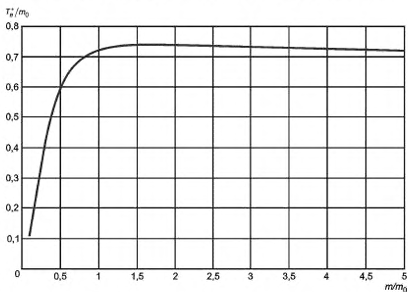
Рисунок A.21 — Взаимосвязь с T_e^*/m_0 для плана испытаний A.7
