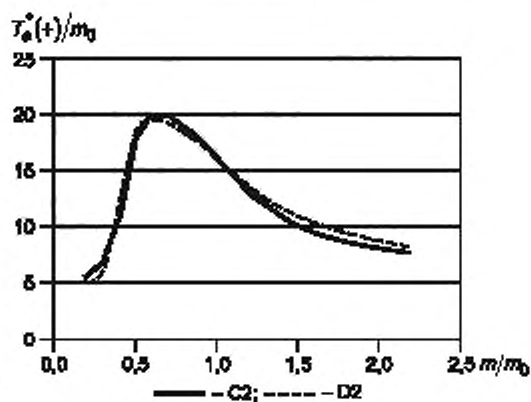
Рисунок D.7 — Зависимость T_e^*(+)/m_0 от m/m_0
