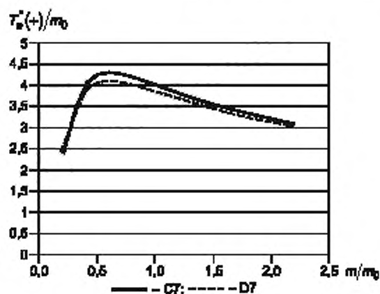
Рисунок D.27 — Зависимость T_e^*(+)/m_0 от m/m_0
