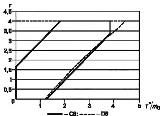
Рисунок D.29 — Линии приемки и отклонения
