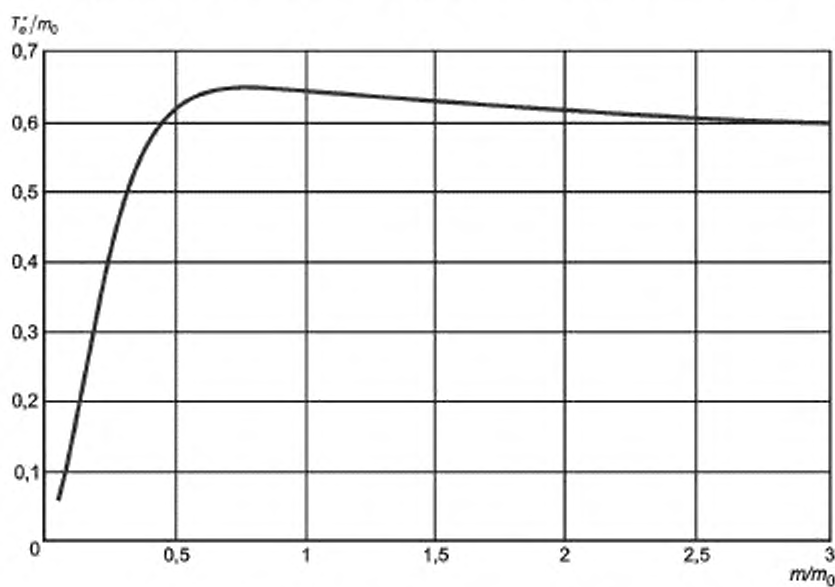
Рисунок А.12 — Взаимосвязь T_g^*/m_0 для плана испытаний А.4
