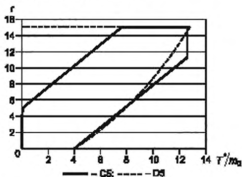
Рисунок D.17 — Линии приемки и отклонения
