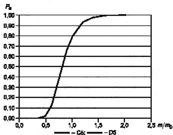
Рисунок D.20 — Оперативная характеристика P_a
