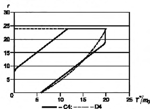
Рисунок D.13 — Линии приемки и отклонения
