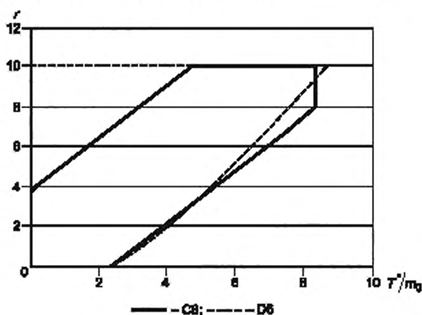
Рисунок D.21 — Линии приемки и отклонения
