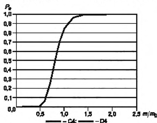
Рисунок D.16 — Оперативная характеристика P_a
