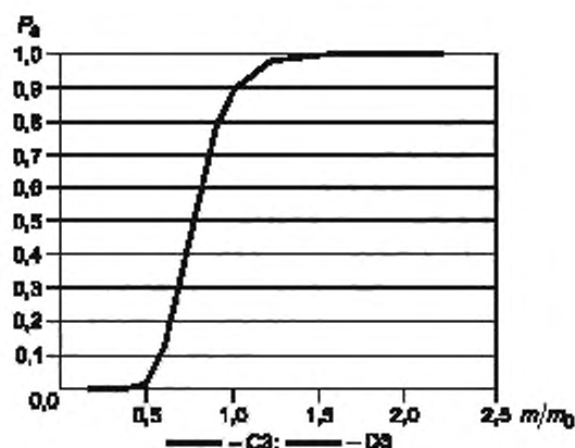
Рисунок D.12 — Оперативная характеристика P_g
