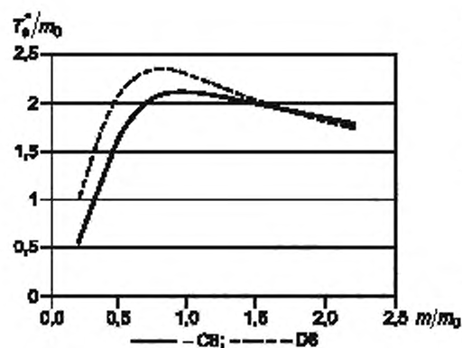
Рисунок D.30 — Зависимость T_e^*/m_0 от m/m_0
