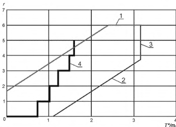
Рисунок Е.1 — Пример плана последовательных испытаний А.3: \alpha = \beta = 10\% , D = 3 , m_0 = 1,11 \cdot 10^6 ч, в координатах \left(\frac{T^*}{m_0}, r\right)
