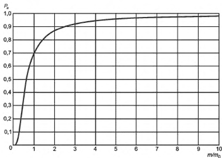
Рисунок A.20 — Кривая оперативной характеристики для плана испытаний A.7
