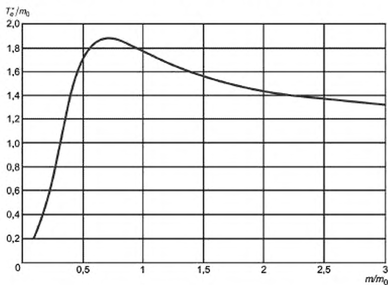
Рисунок A.9 — Взаимосвязь T_a^*/m_0 для плана испытаний A.3
