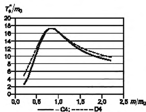
Рисунок D.14 — Зависимость T_e^*/m_0 от m/m_0
