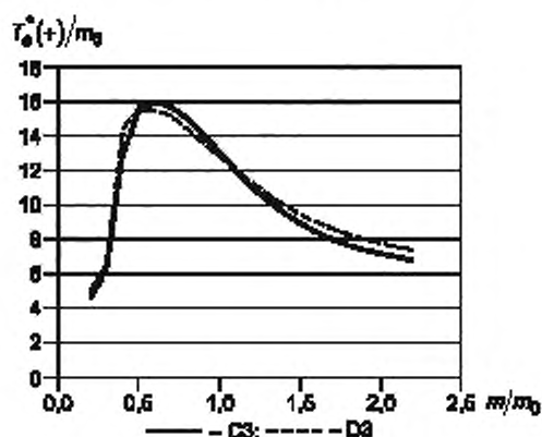
Рисунок D.11 — Зависимость T_e^*(+)/m_0 от m/m_0
