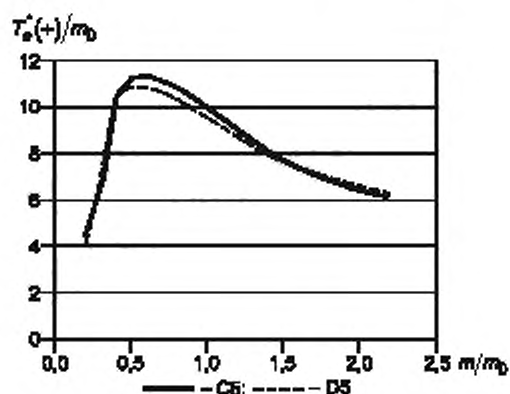
Рисунок D.19 — Зависимость T_e^*(+)/m_0 от m/m_0
