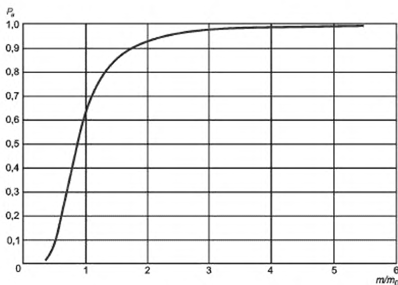
Рисунок A.23 — Кривая оперативной характеристики для плана испытаний A.8
