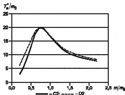
Рисунок D.6 — Зависимость T_e^*/m_0 от m/m_0
