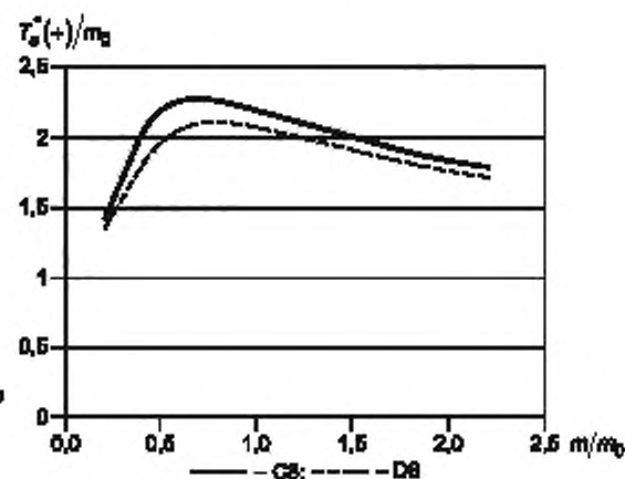
Рисунок D.31 — Зависимость T_e^*(+)/m_0 от m/m_0
