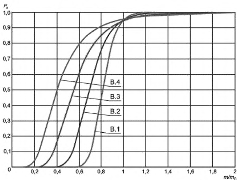
Рисунок В.1 — Кривые оперативных характеристик для планов испытаний В.1, В.2, В.3 и В.4
