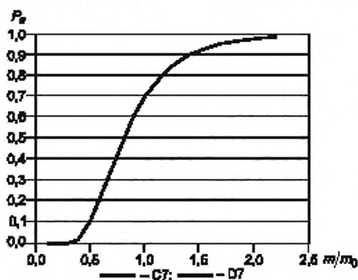
Рисунок D.28 — Оперативная характеристика P_a
