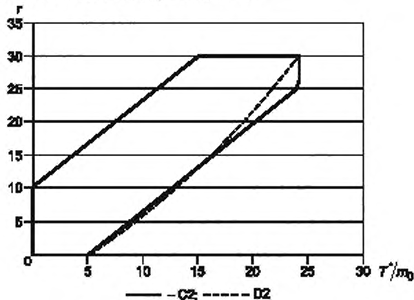
Рисунок D.5 — Линии приемки и отклонения
