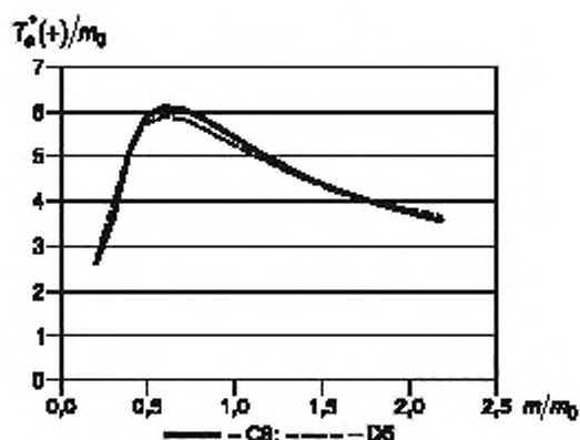
Рисунок D.23 — Зависимость T_e^*(+)/m_0 от m/m_0
