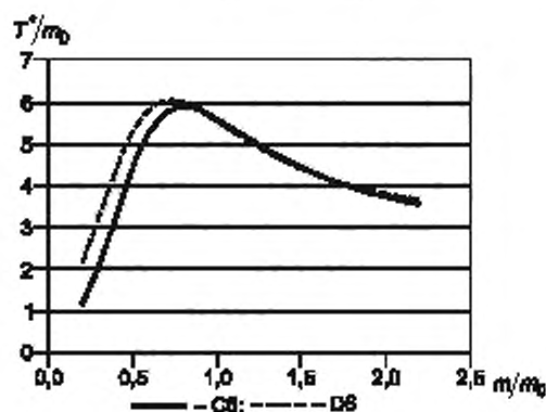
Рисунок D.22 — Зависимость T_e^*/m_0 от m/m_0
