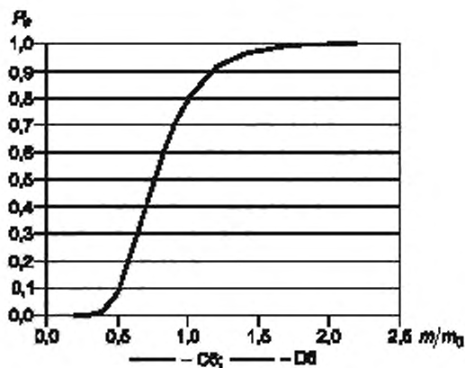
Рисунок D.24 — Оперативная характеристика P_a
