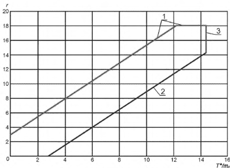
Рисунок F.1 — Пример графика SPRT
