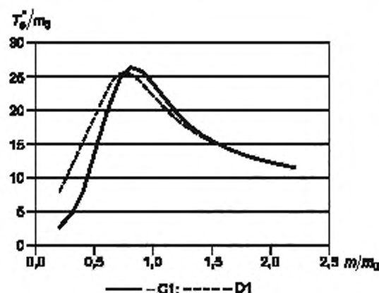
Рисунок D.2 — Зависимость T_e^*/m_0 от m/m_0
