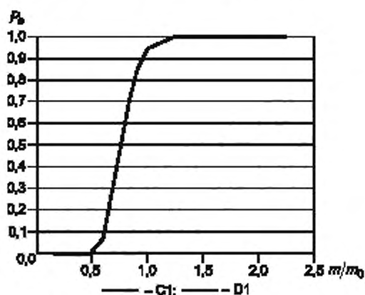
Рисунок D.4 — Оперативная характеристика P_a
