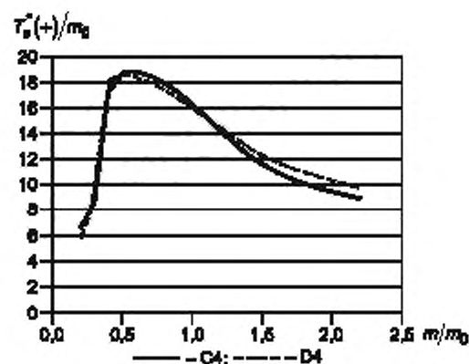
Рисунок D.15 — Зависимость T_e^*(+)/m_0 от m/m_0
