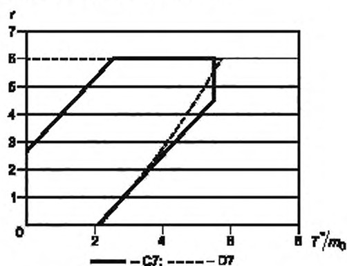
Рисунок D.25 — Линии приемки и отклонения
