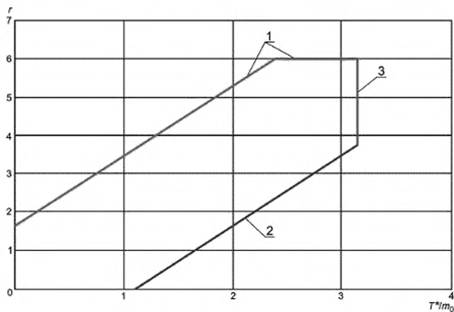
Рисунок А.7 — Линии приемки и отклонения для плана испытаний А.3
