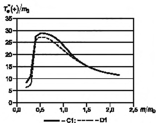
Рисунок D.3 — Зависимость T_e^*(+)/m_0 от m/m_0
