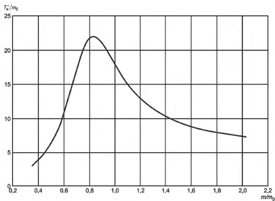
Рисунок А.3 — Взаимосвязь T'_a/m_0 для плана испытаний А.1
