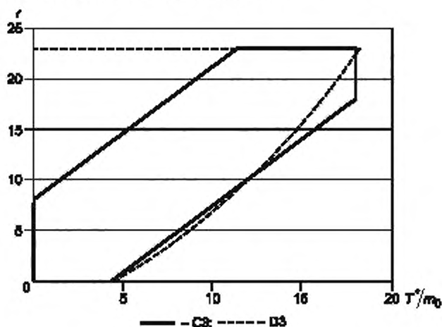
Рисунок D.9 — Линии приемки и отклонения
