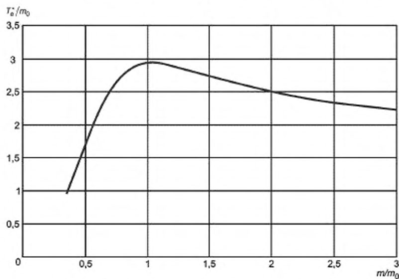
Рисунок A.24 — Взаимосвязь с T_e^*/m_0 для плана испытаний A.8
