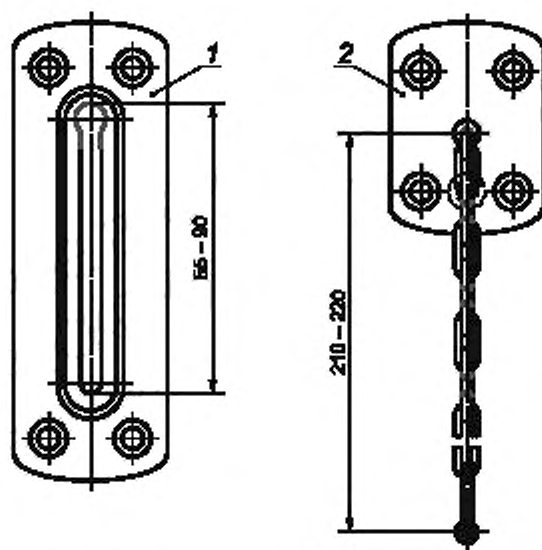
1 — запорная планка, 2 — основание
