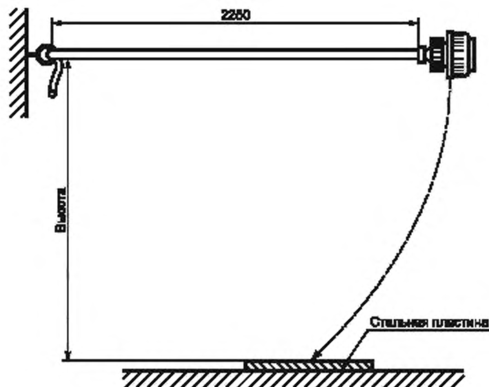
Рисунок 1 — Пример монтажа соединителя
