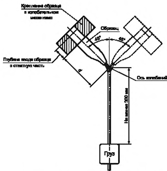
Рисунок 2 — Схема перемещения испытываемого образца неразъемного соединителя во время испытания прочности на изгиб
