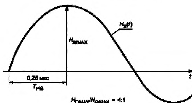
Рисунок А.2б — Моделирование нарастания магнитного поля последующих ударов молнии (0,25/100 мкс) при помощи затухающих колебаний частотой 1 МГц (многократные импульсы 0,2/0,5 мкс)
