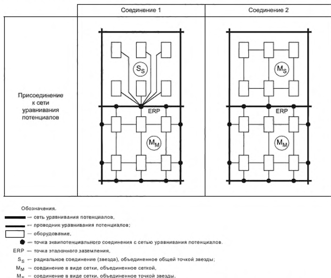
Рисунок 10 — Комбинации способов присоединения проводящих частей внутренних систем к сети уравнивания потенциалов
