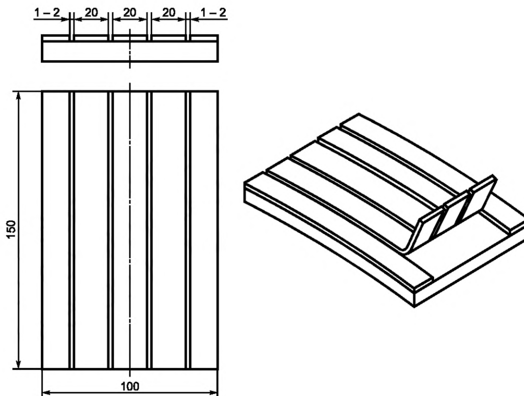
Рисунок К.3 — Испытательный образец для определения адгезии методом отслаивания под углом ( 90 \pm 10 )°
