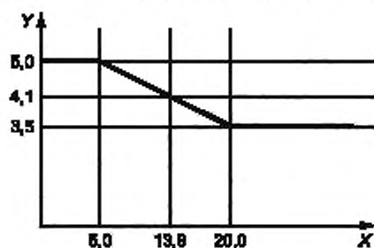
Рисунок 7 — Максимальное замедление
