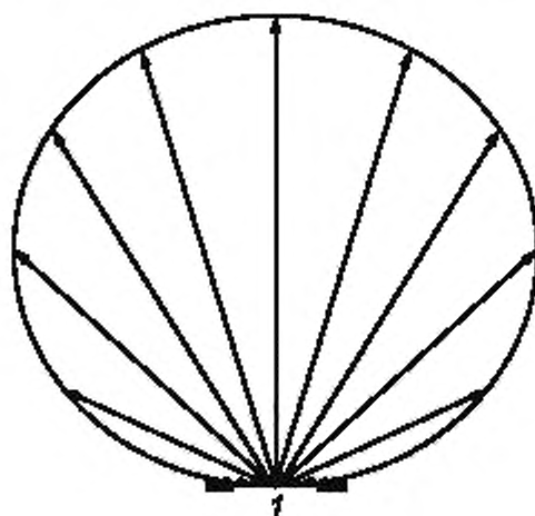
1 — отражатель
