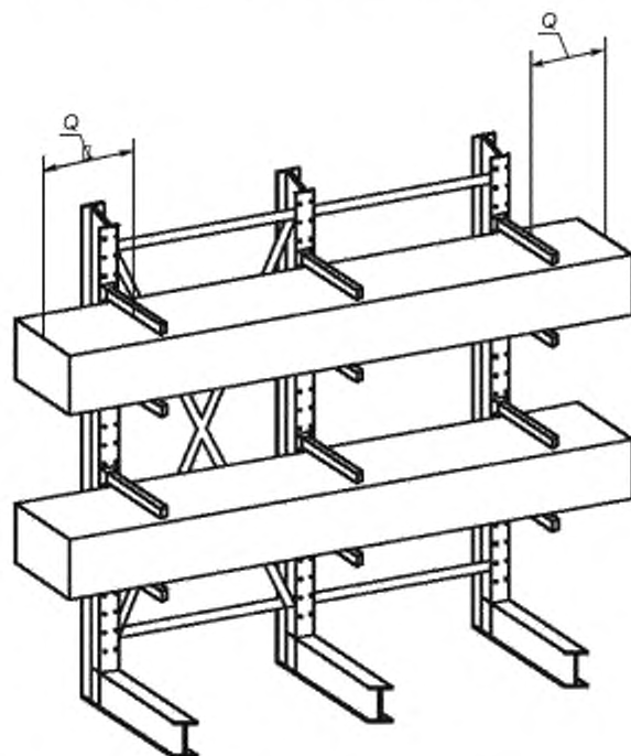
Рисунок 12 — Размещение грузов на консольных стеллажах
