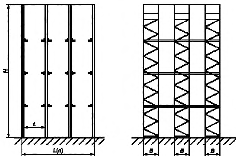
Рисунок 2 — Общий вид набивного (глубинного) стеллажа
