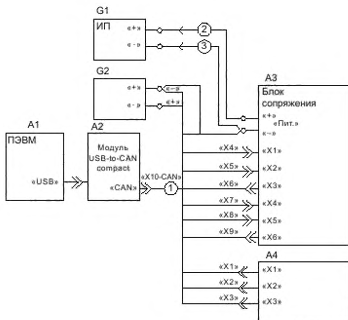
A1 — ПЭВМ; A2 — модуль USB-to-CAN, A3 — блок сопряжения; A4 — испытываемая УСВ. G1 — источник питания, G2 — испытательный генератор импульсных помех в бортовой сети автотранспортных средств;
