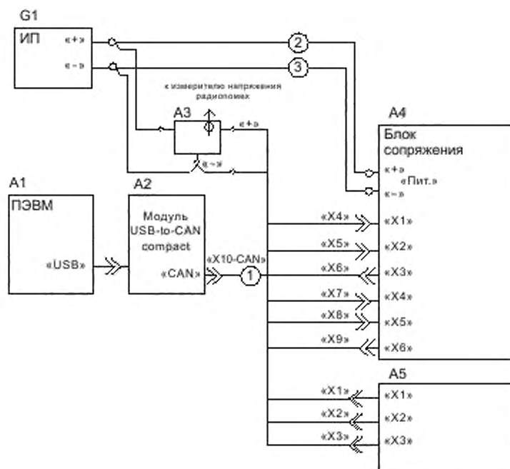
А1 — ПЭВМ; А2 — модуль USB-to-CAN; А3 — V-образный эквивалент сети (см. таблицу 2); А4 — блок сопряжения, А5 — испытываемая УСВ; G1 — источник питания; L1 — катушка индуктивности с воздушным сердечником, рассчитанная на ток до 5 А; P1 — осциллограф; 1 — кабель, 2, 3 — провод ML-4G
