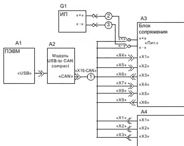
A1 — ПКВМ; A2 — модуль USB-to-CAN; A3 — блок сопряжения; A4 — испытуемая УСВ; G1 — источник питания; 1 — кабель, 2, 3 — провод ML-4G
