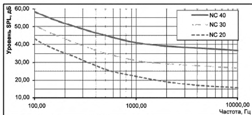
Рисунок 4 — Спектральная плотность окружающего шума
