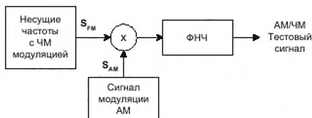
Рисунок 14 — Блок-схема генерации тестовых сигналов на основе набора синусов с AM/ЧМ модуляцией
