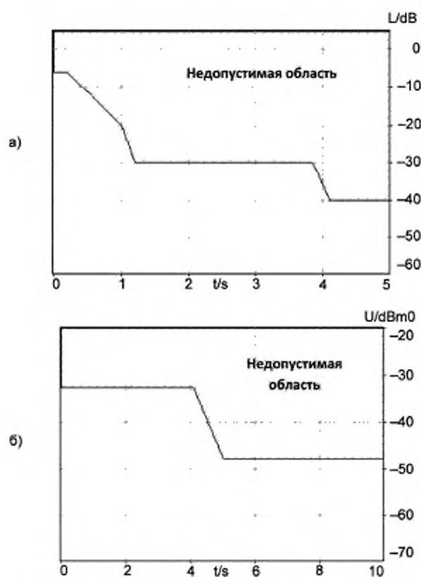
Рисунок 8 — Зависимость степени подавления экосигналов L и уровня экосигналов U от времени
