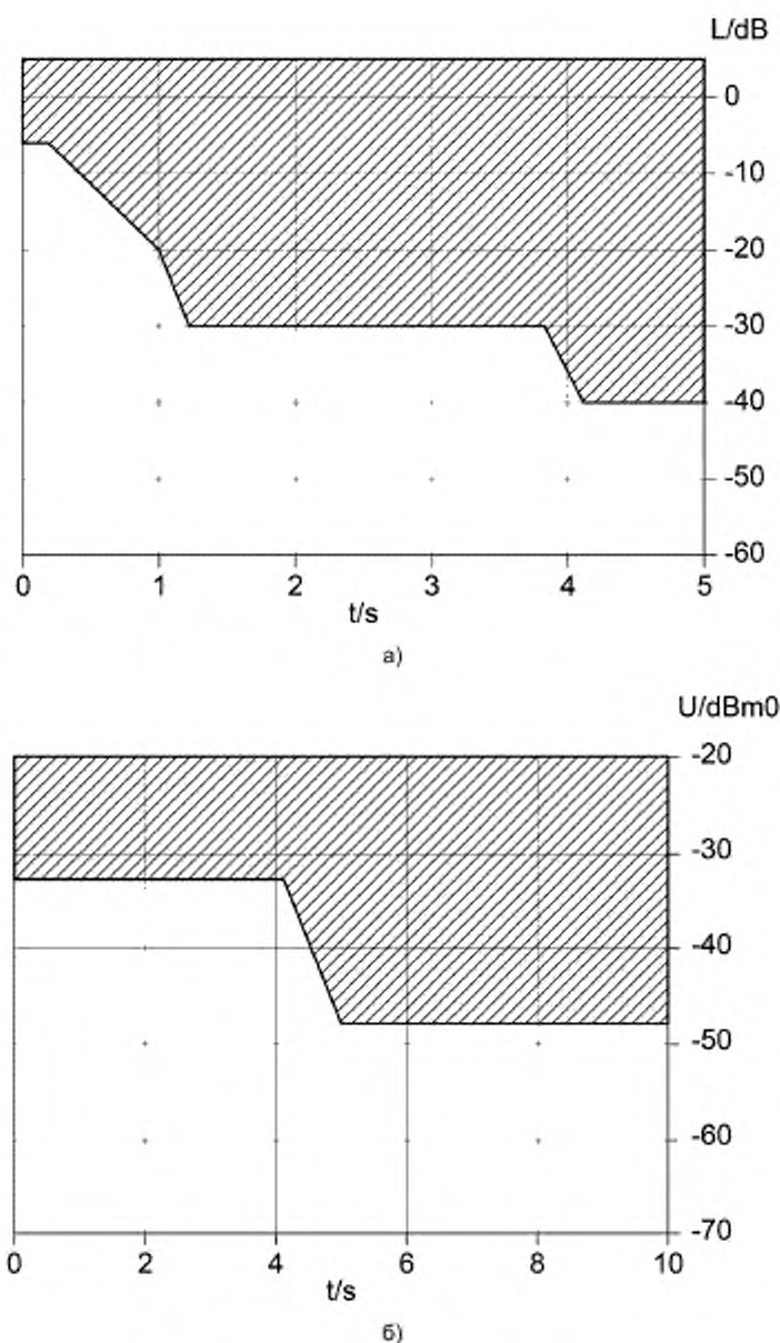
Рисунок И.1 — Зависимость степени подавления эхосигналов L и уровня эхосигналов U от времени
