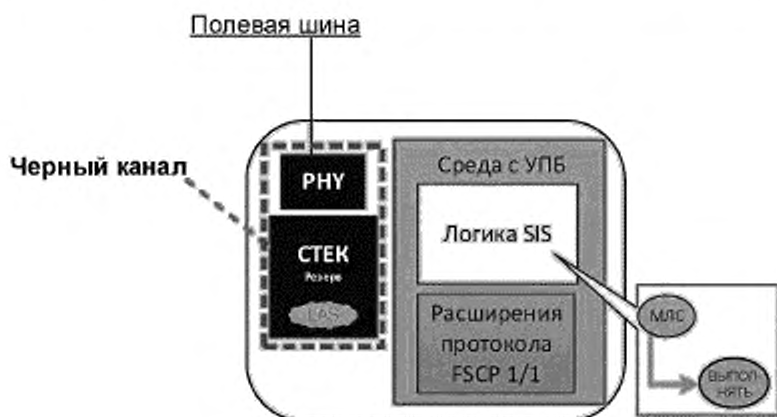
Рисунок 9 — Устройство Н1 с FSCP 1/1
