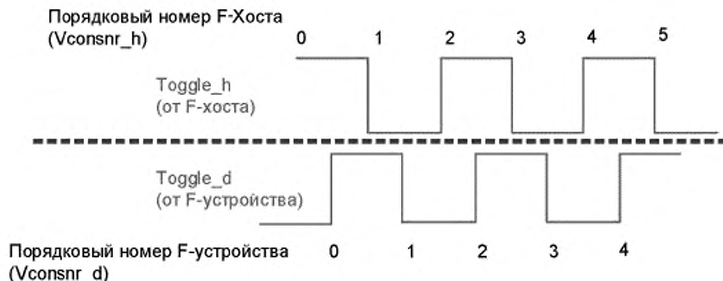
Рисунок 23 — Функция бита переключателя
