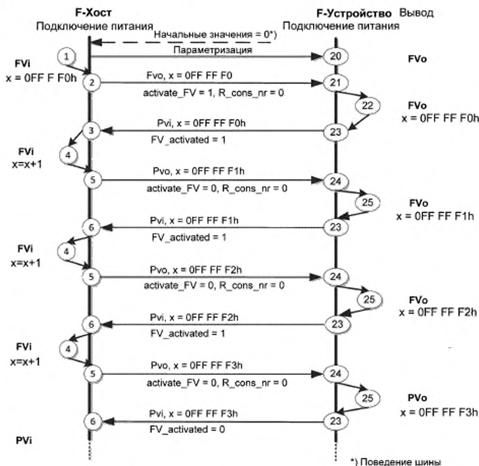
Рисунок 30 — Взаимодействие F-хоста / F-устройства во время запуска
