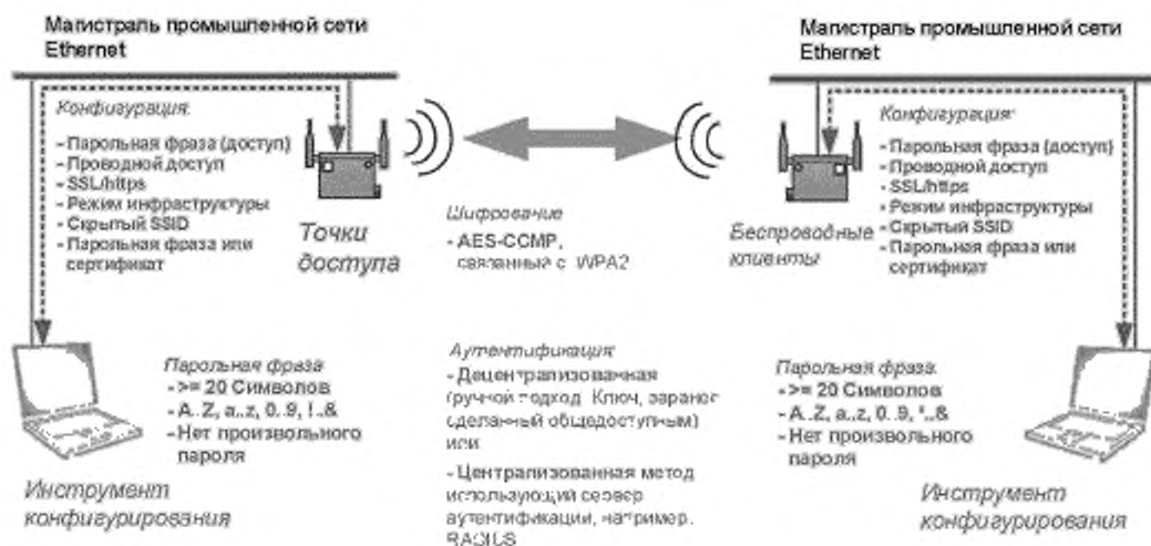
Рисунок 84 — Защита для WLAN сетей
