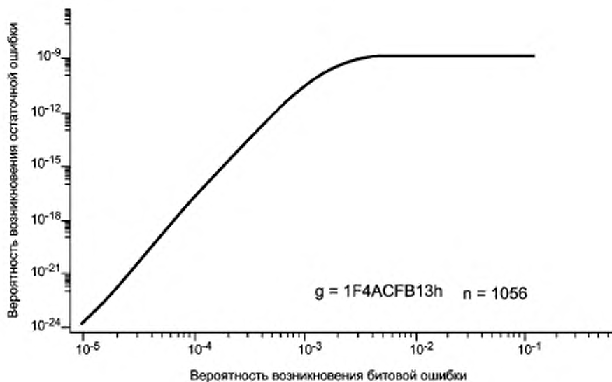
Рисунок 82 — Годность 32-битового полинома для 132 октетов
