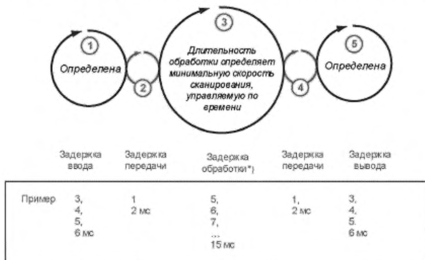
Рисунок 73 — Упрощенная модель типового времени реакции
