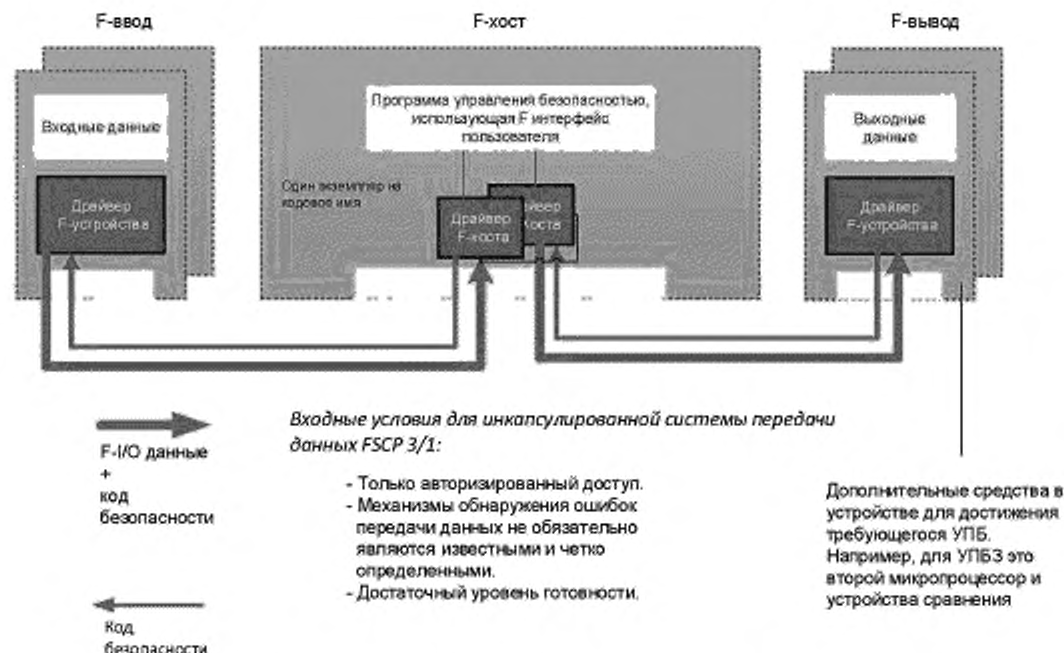
Рисунок 17 — Структура коммуникаций FSCP 3/1
