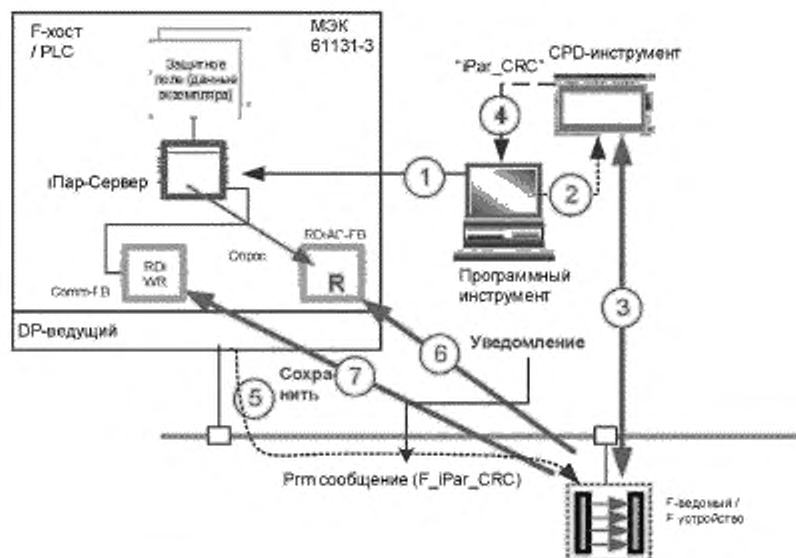
Рисунок 66 — Механизм iPar-сервера (ввод в эксплуатацию)
