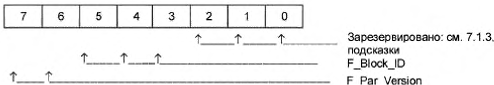
Рисунок 48 — F_Prm_Flag2
