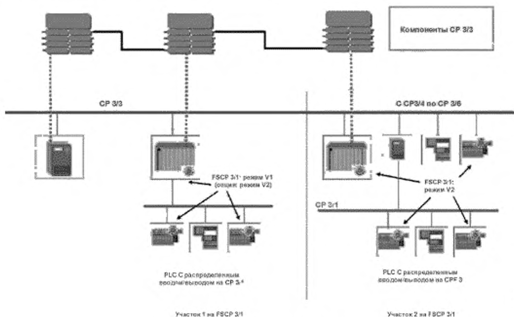
Рисунок 5 — Режимы коммуникаций безопасности
