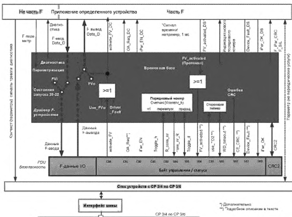
Рисунок 19 — Интерфейсы драйвера F-устройства
