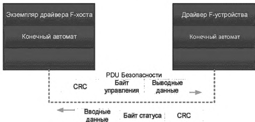
Рисунок 27 — Коммуникационная связь уровня безопасности
