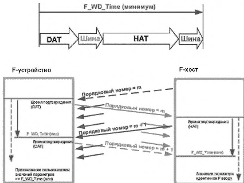
Рисунок 76 — Временные секции, формирующие F_WD_Time профиля FSCP 3/1
