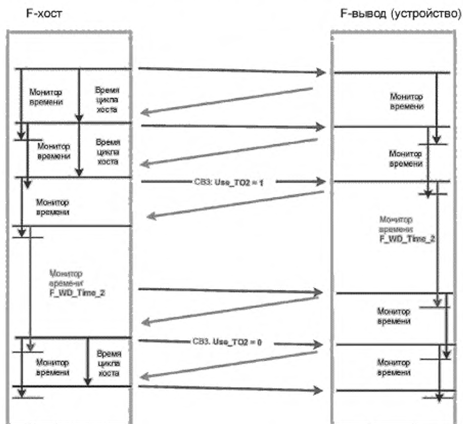
Рисунок 39 — Расширенное время сторожевого таймера по запросу
