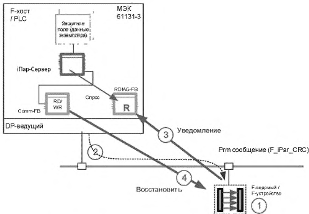
Рисунок 67 — Механизм іпар-сервера (наприклад, заміна F-устройства)
