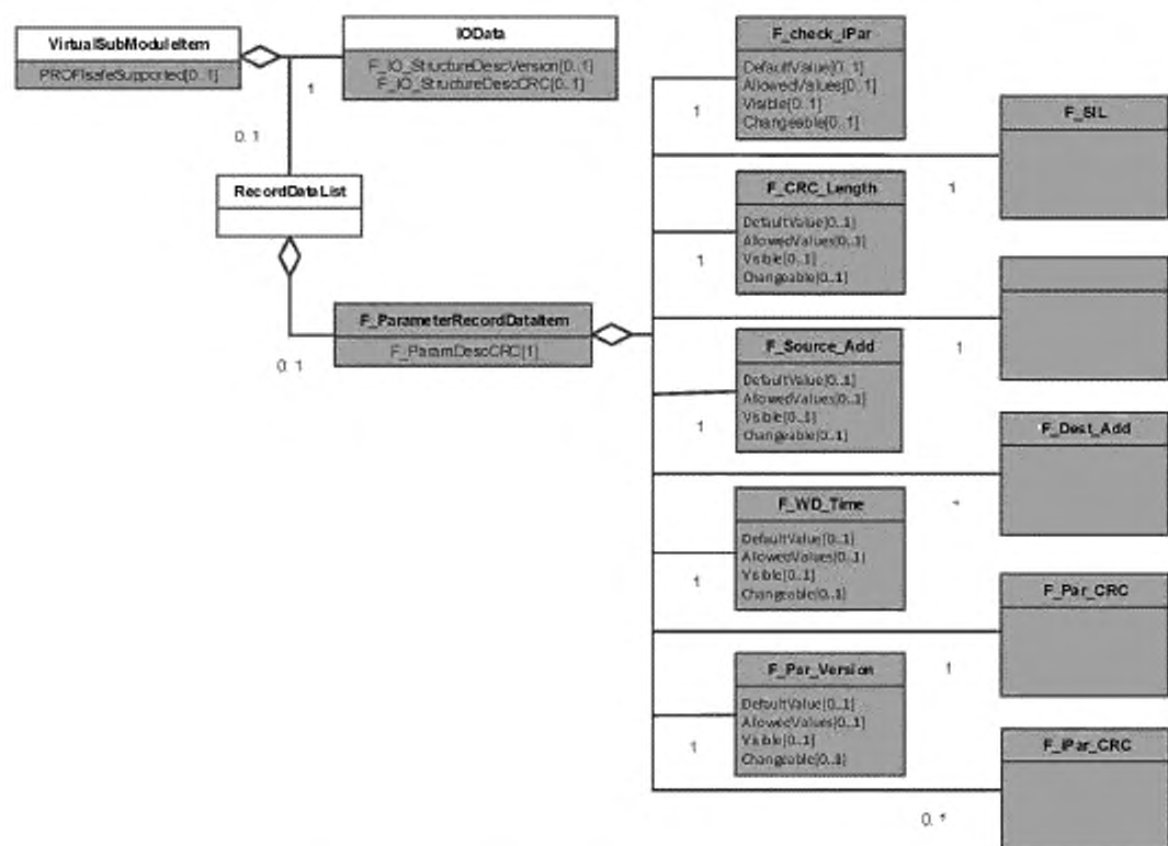
Рисунок 53 — Расширение F-параметра в спецификации GSDML
