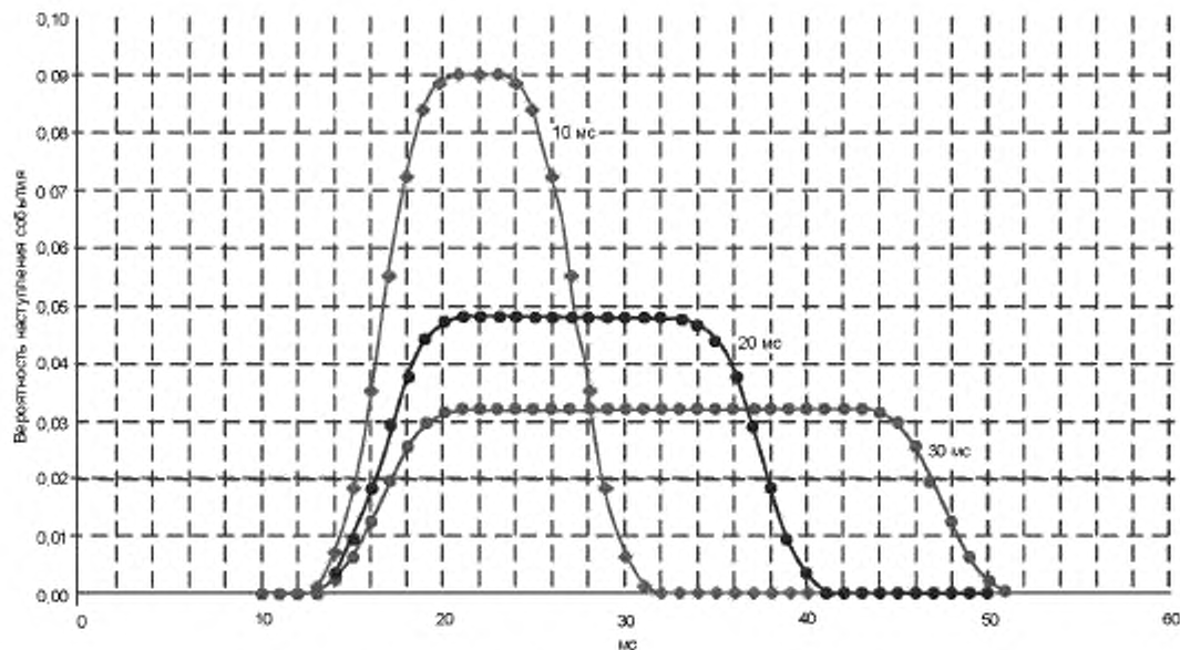
Рисунок 74 — Распределения частот типового времени реакции модели
