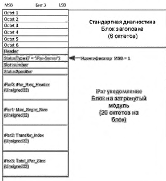
Рисунок 68 — Кодирование запроса iPar-сервера («модель статуса»)
