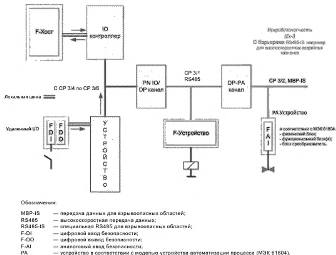
Рисунок 12 — Полные пути передачи данных безопасности
