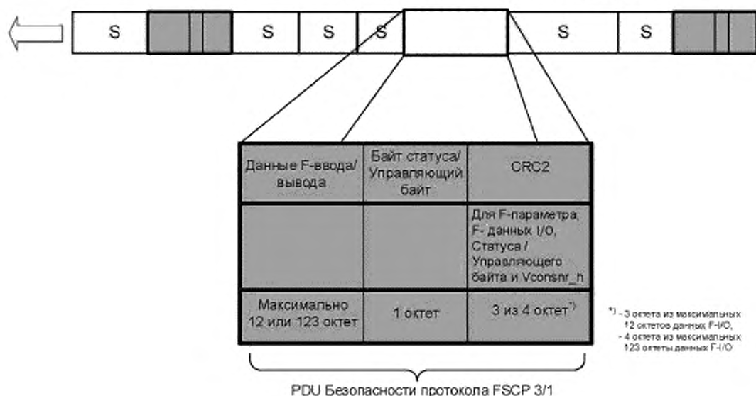
Рисунок 20 — PDU безопасности для CPF 3
