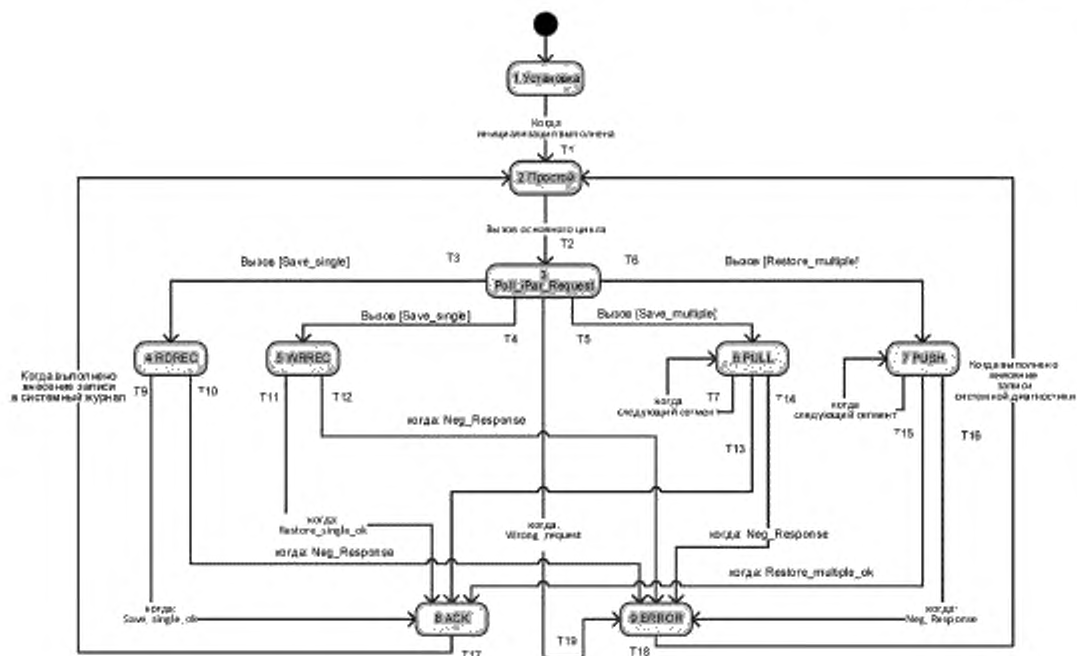
Рисунок 71 — Диаграмма состояний iPAR-сервера
