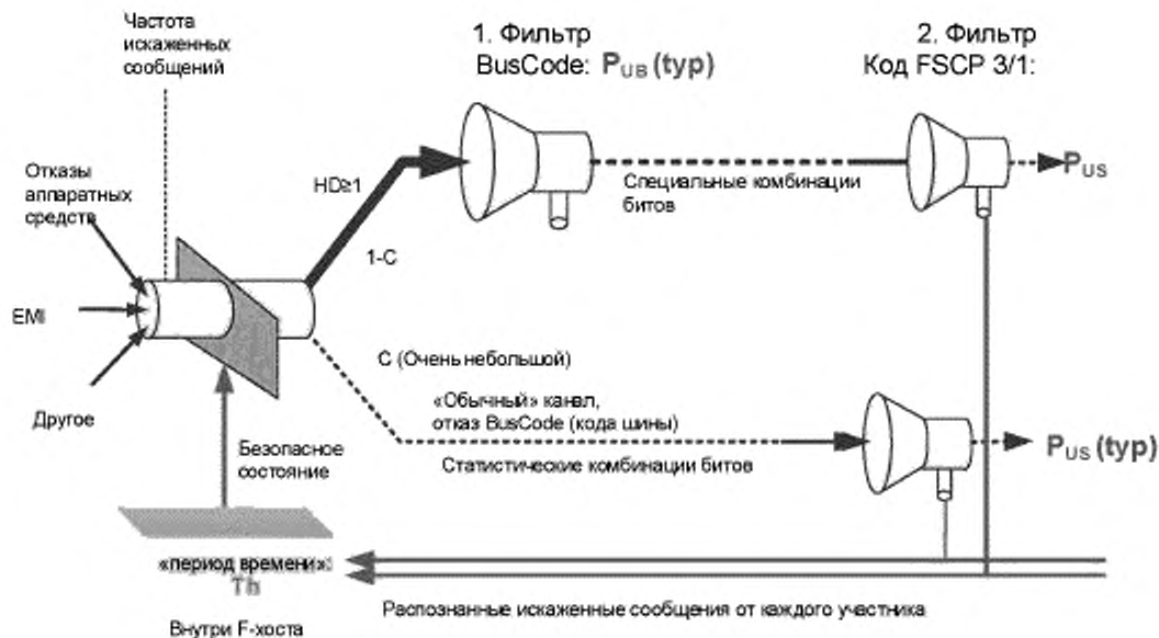
Рисунок 83 — Контроль искаженных сообщений
