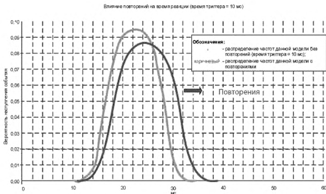
Рисунок 77 — Кривая распределения времени реакции с повторениями сообщений
