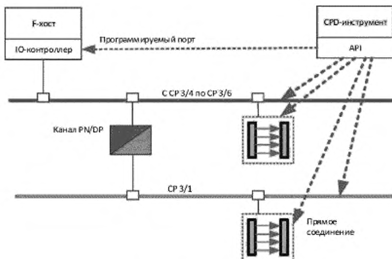
Рисунок 65 — Интеграция системы CPD-инструментов
