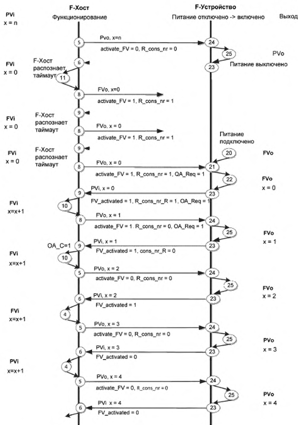
Рисунок 32 — Взаимодействие F-хоста / F-устройства с задержкой включения питания
