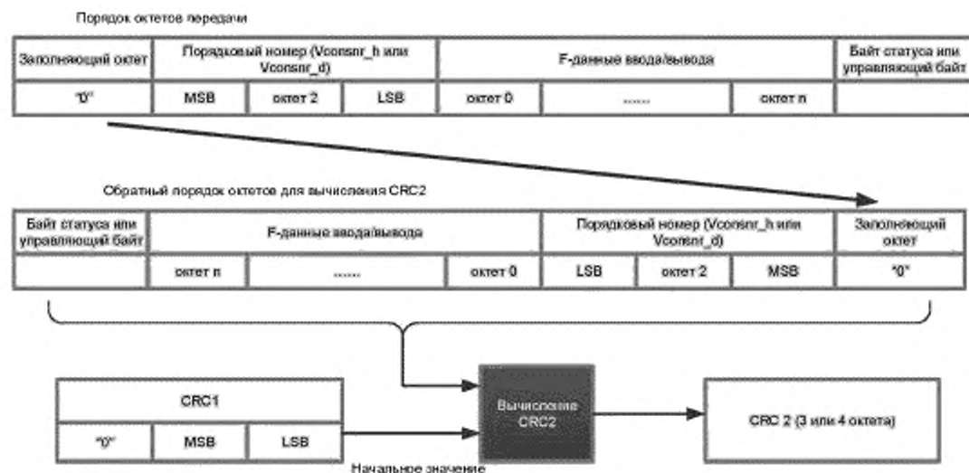
Рисунок 26 — Подробности вычисления CRC2 (обратный порядок)
