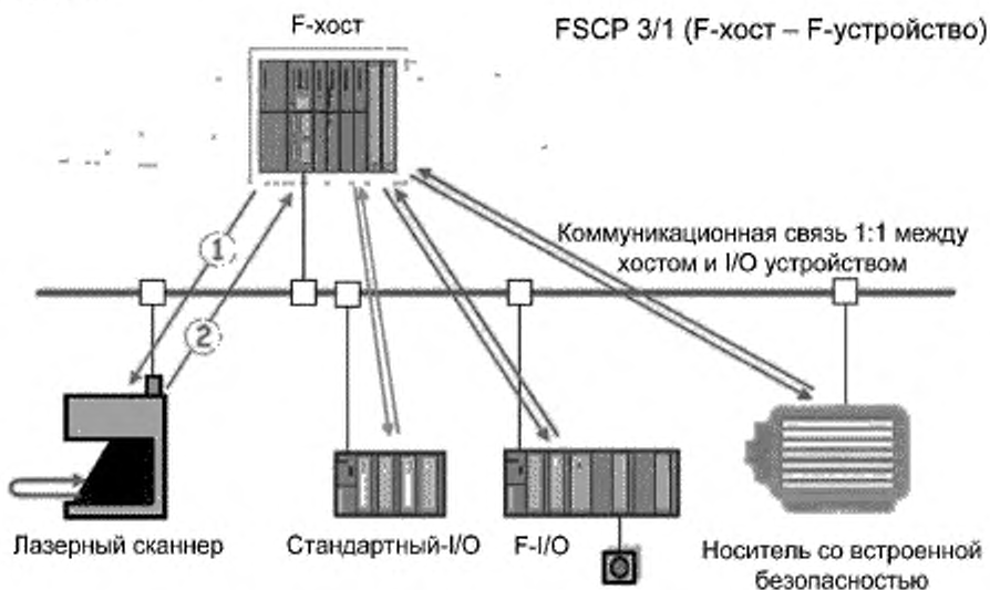
Рисунок 6 — Стандартная система передачи CPF 3
