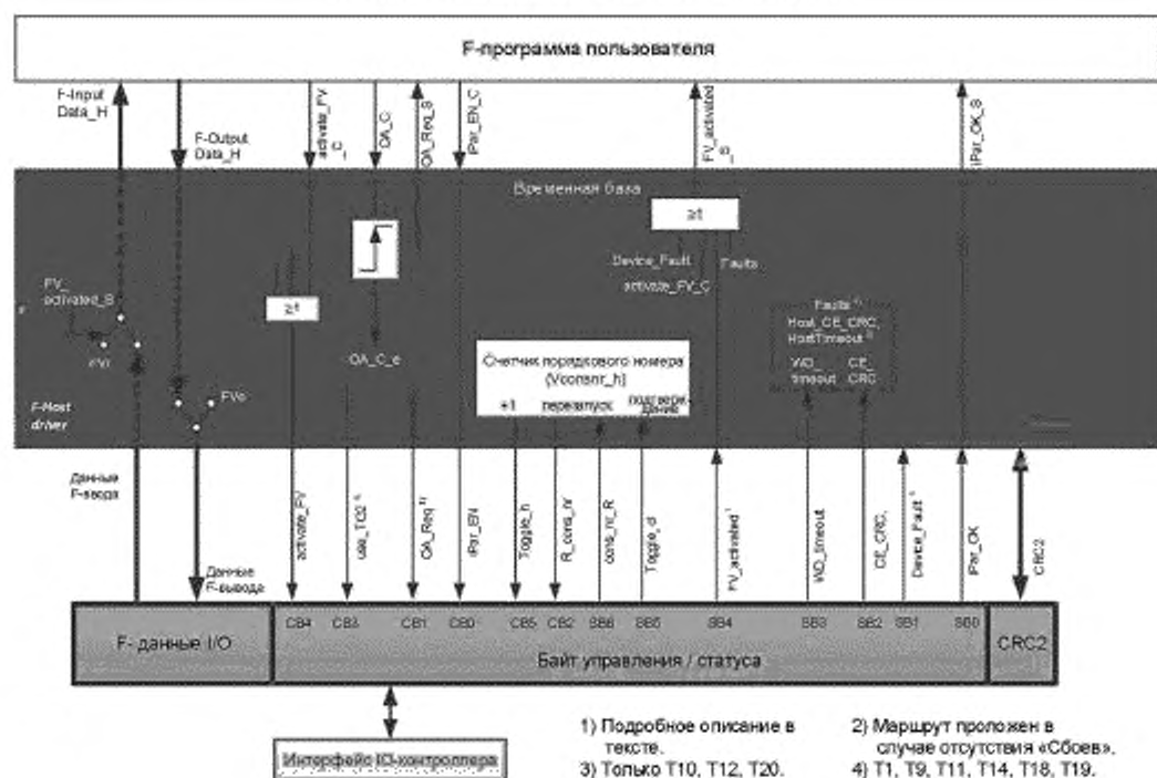
Рисунок 18 — F-интерфейс пользователя для экземпляров драйвера F-хоста
