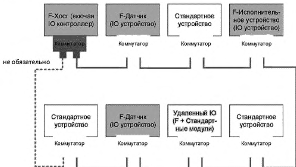
Рисунок 10 — Линейная структура шины
