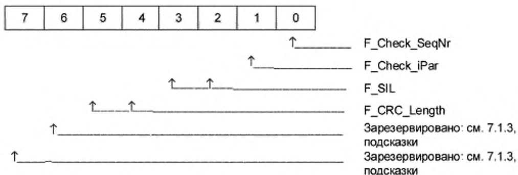
Рисунок 43 — F_Prm_Flag1
