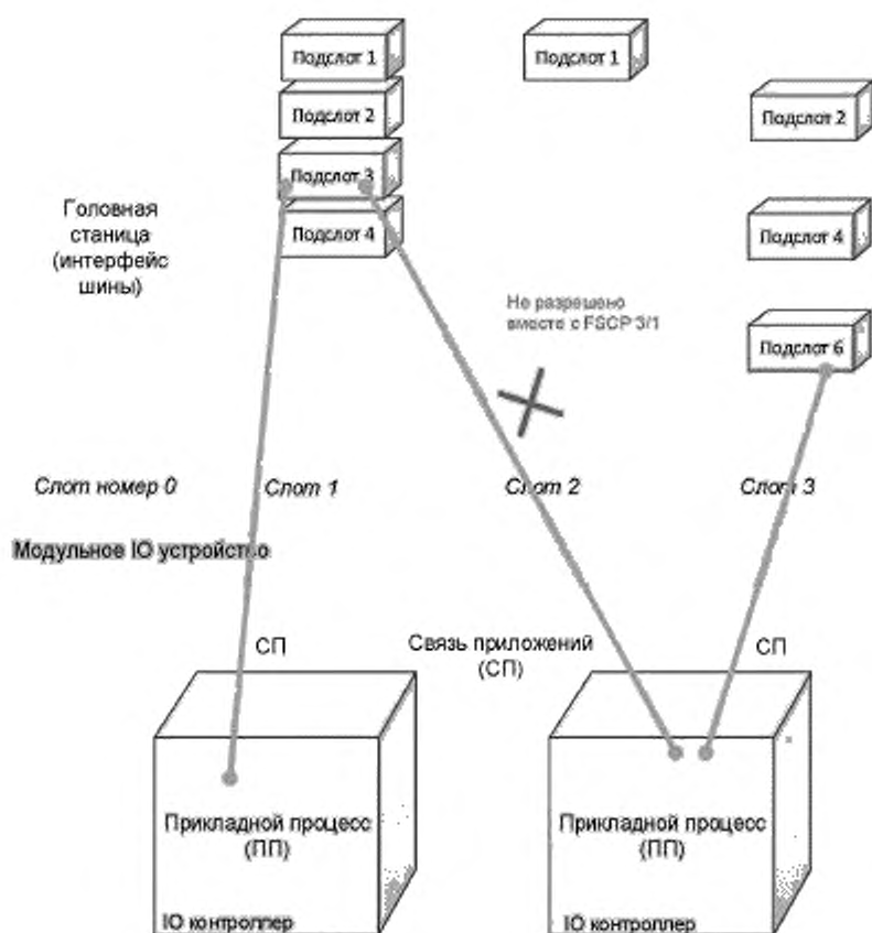
Рисунок 14 — Связи приложений модульного устройства
