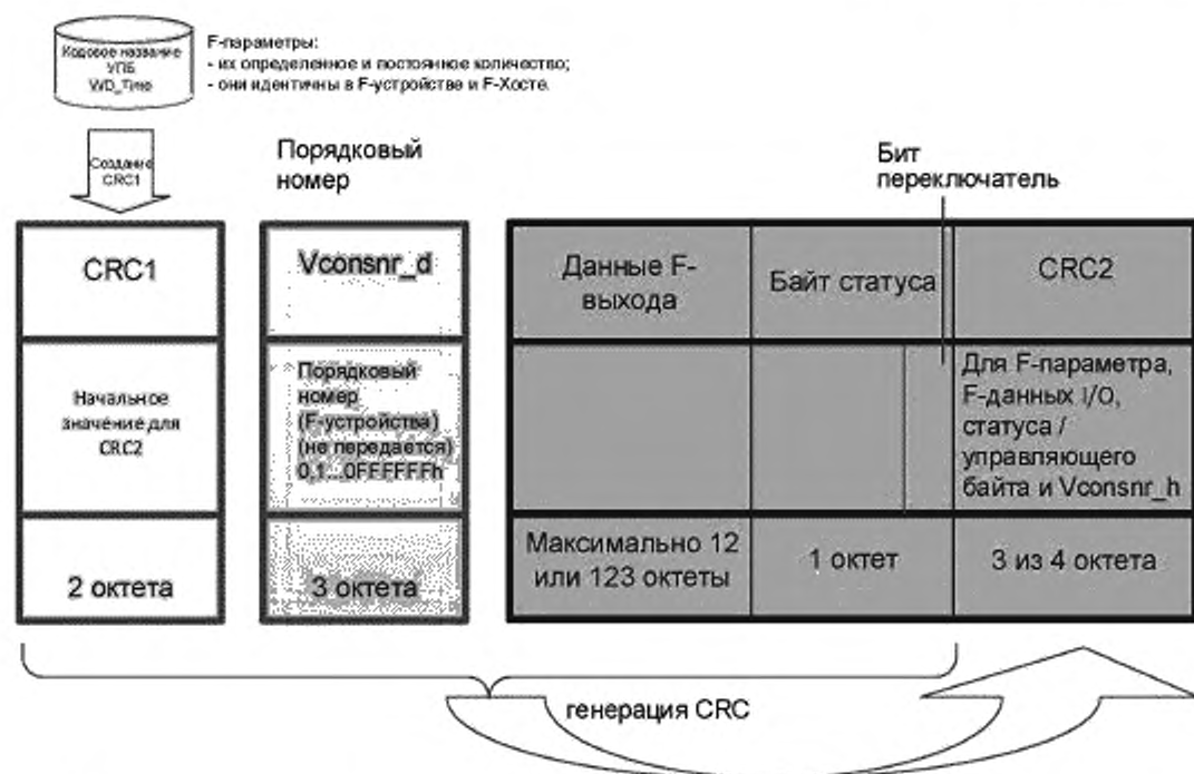
Рисунок 25 — Генерация CRC2 (вывод F-хоста)
