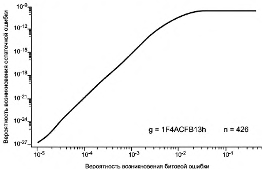
Рисунок 81 — Годность 32-битового полинома для 52 октетов
