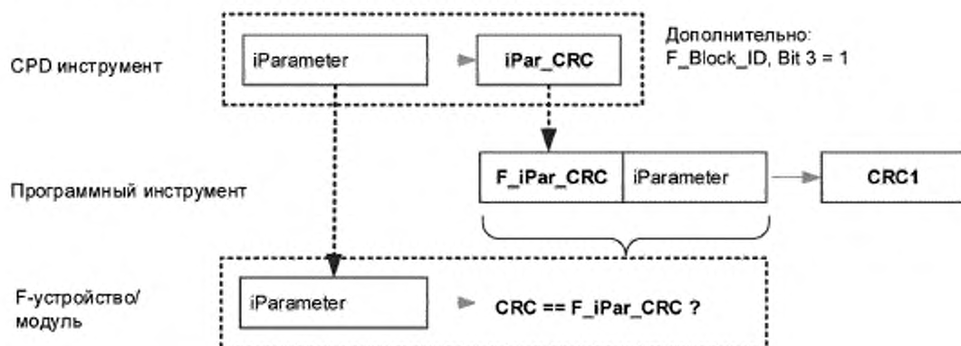
Рисунок 54 — CRC1, включая iPar_CRC
