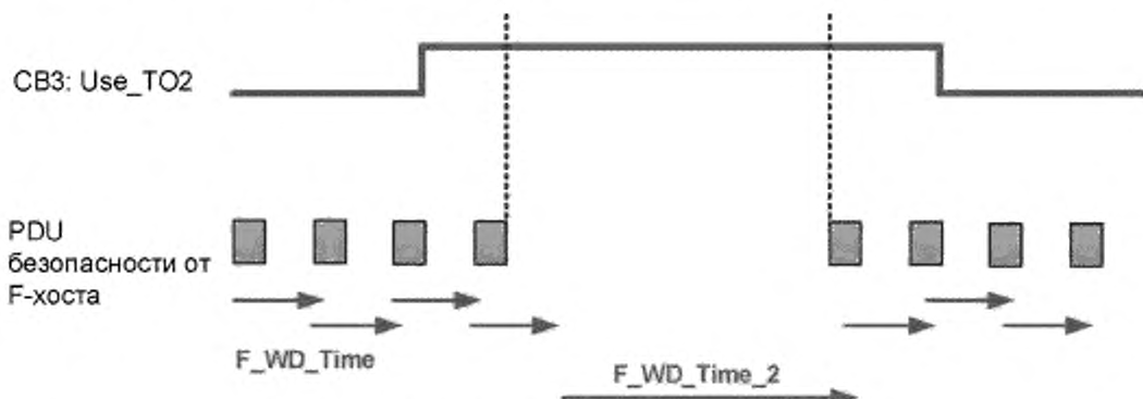
Рисунок 42 — Эффект F_WD_Time_2
