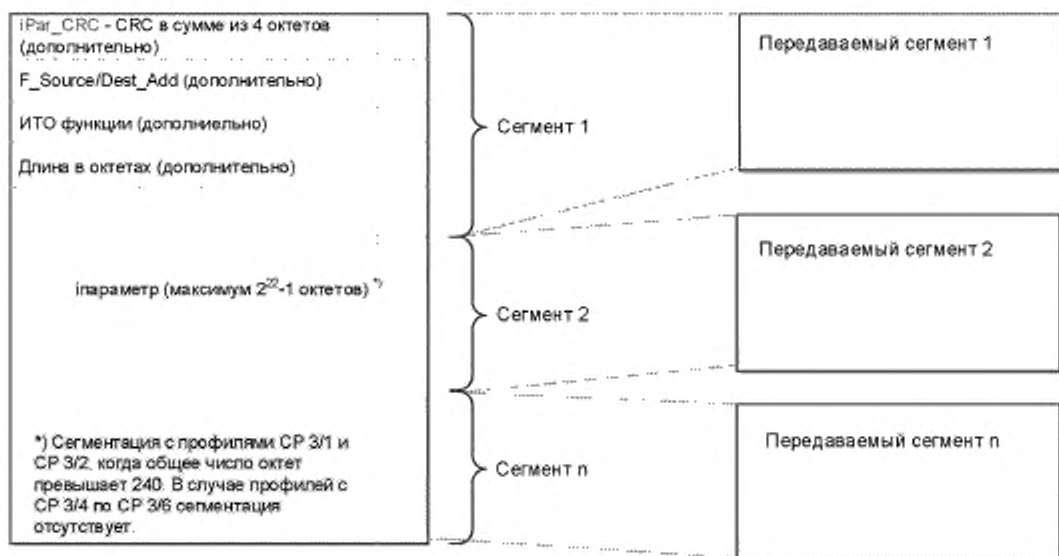
Рисунок 52 — Блок iпараметров
