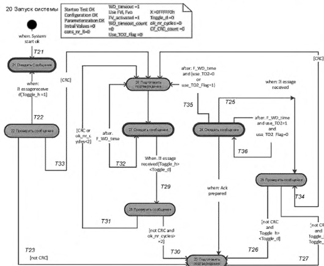
Рисунок 29 — Диаграмма состояний F-устройства
