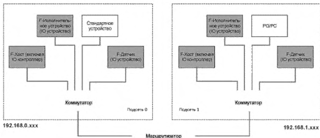
Рисунок 11 — Пересечение границ сети с маршрутизаторами
