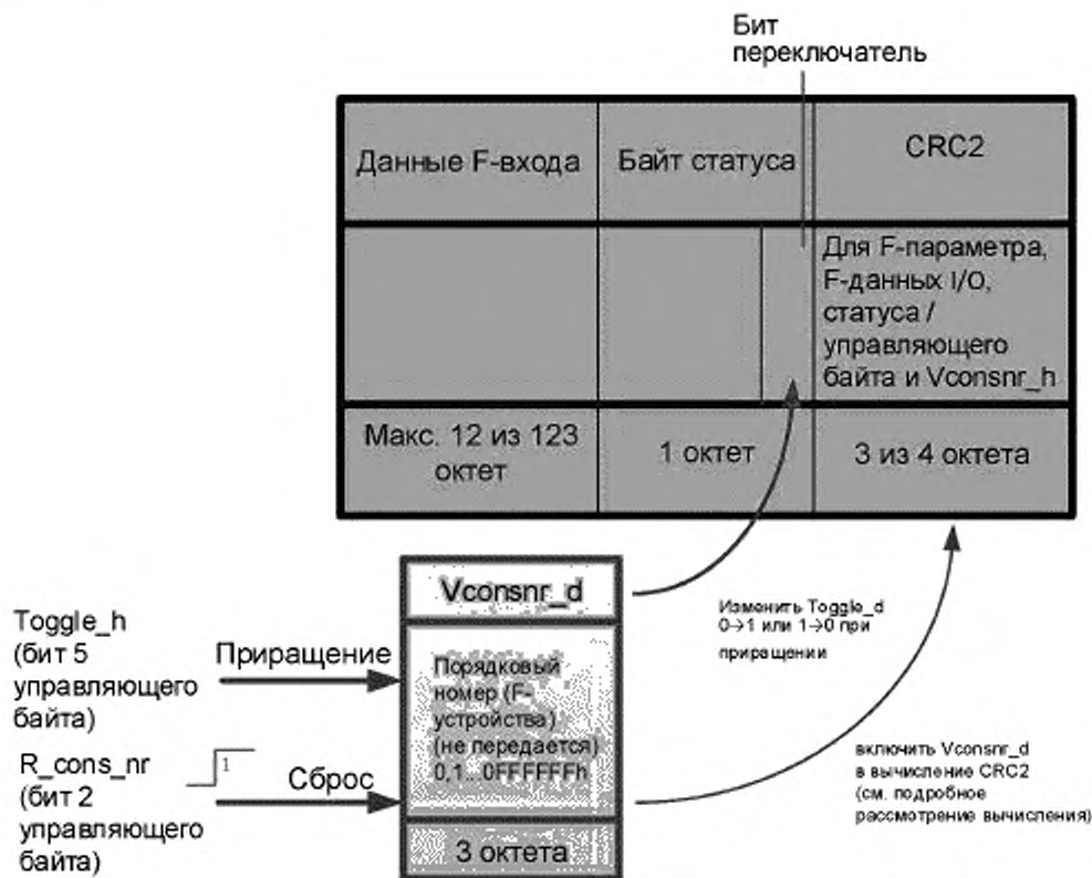
Рисунок 24 — Порядковый номер F-устройства
