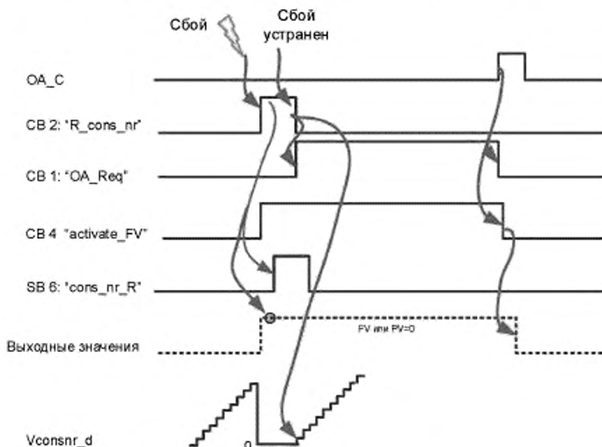
Рисунок 36 — Влияние сигнала сброса счетчика
