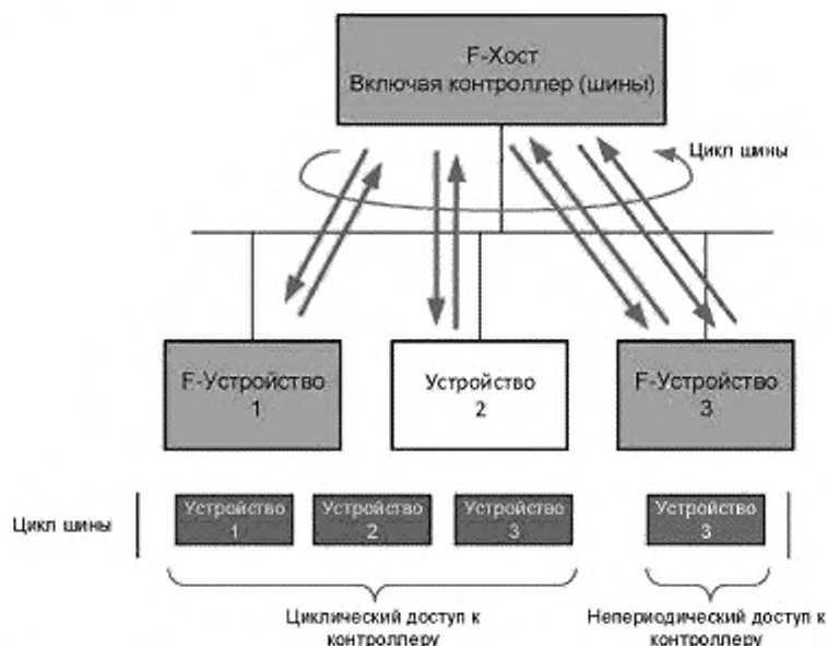
Рисунок 3 — Базовые предварительные условия для коммуникаций в FSCP 3/1
