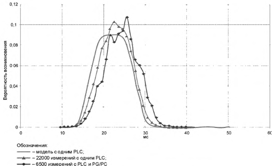
Рисунок А.2 — Распределение частот измеренного времени реакции
