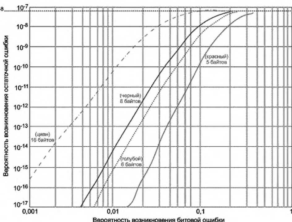
Рисунок 80 — Вероятности возникновения остаточной ошибки для 24-битового полинома
