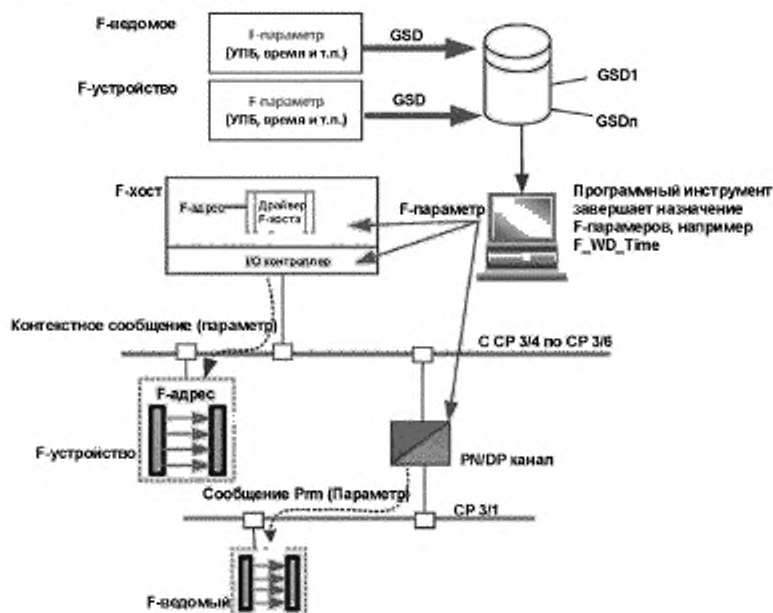
Рисунок 63 — Назначение F-параметров простым F-устройствам и F-ведомым устройствам
