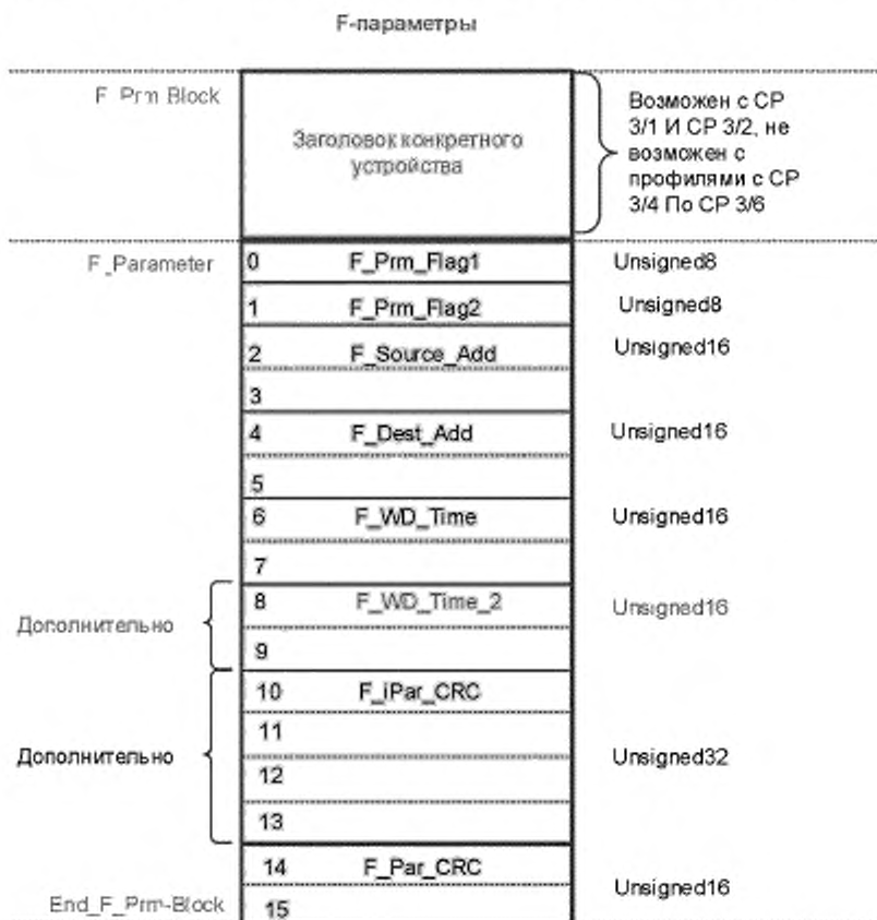
Рисунок 51 — F-параметр
