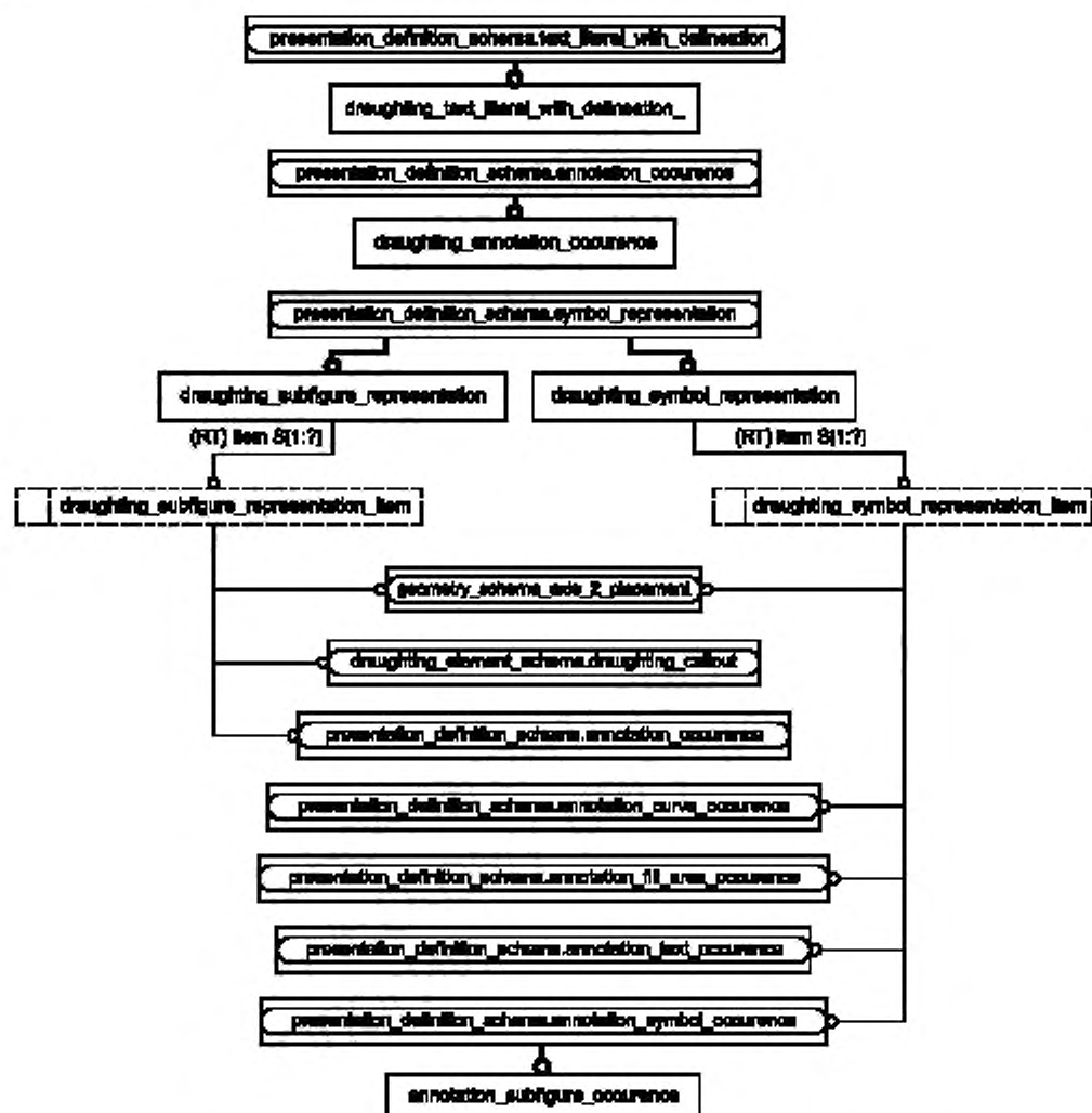
Рисунок D.2 – EXPRESS-G диаграмма схемы aisc_draughting_annotation. Диаграмма 2 из 2
