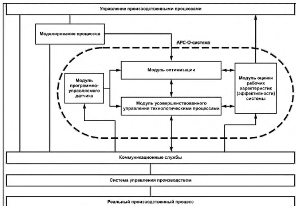
Рисунок 2 — Функциональная архитектура APC-O-системы
