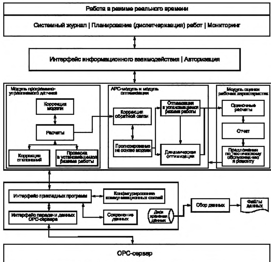
Рисунок А.1 — Типовой пример интеграции модулей APC-O-системы
