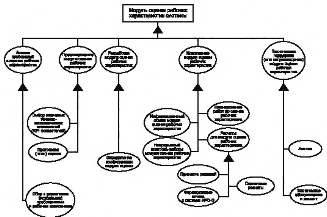
Рисунок 7 — Фазы жизненного цикла модуля оценки рабочих характеристик
