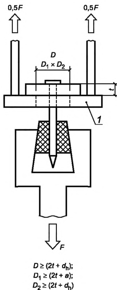
1 — стальная пластина с круглым отверстием (диаметр D ) для гвоздей и винтов и прямоугольным отверстием (длины сторон D_1 и D_2 ) для скоб
