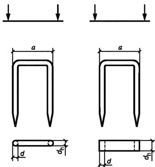
Рисунок 1 — Размеры скобы
