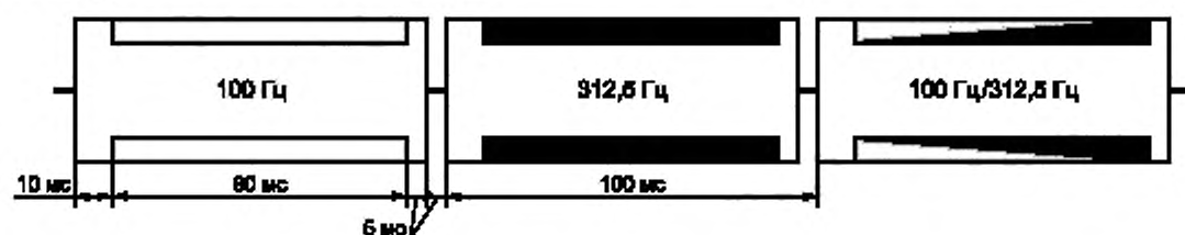
Рисунок 1 — Фрагмент структуры сигнала типа DXXXW
