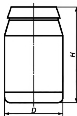
Банка БНЦ Рисунок А.3
