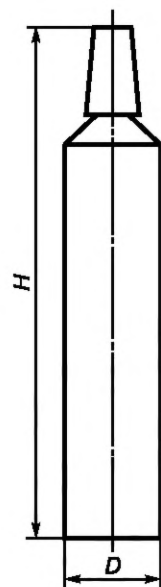
Туба Рисунок А.12
