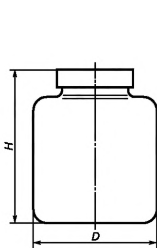
Банка БНЦ Рисунок А.1
