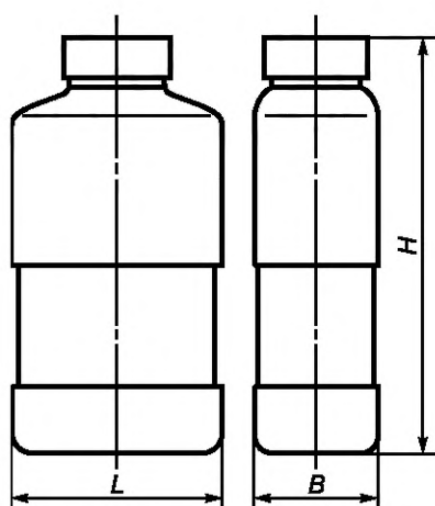
Банка БНП Рисунок А.4
