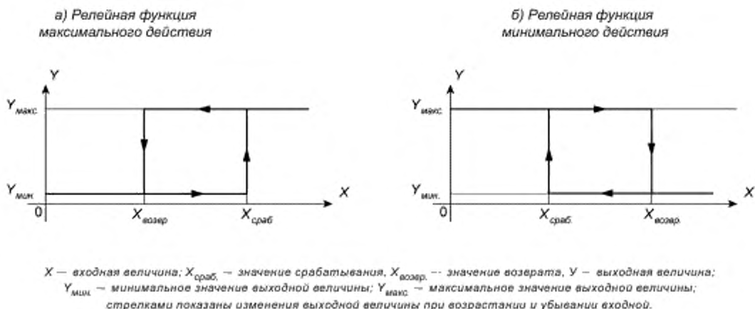
Рисунок 1 — Графики релейных функций одной входной величины
