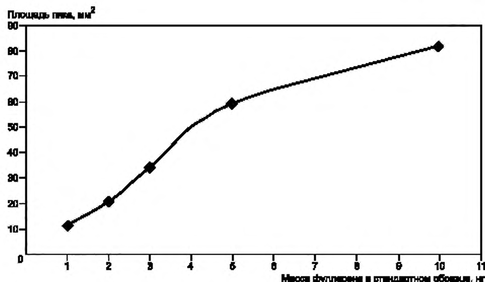
Рисунок Г.3 — Пример градуировочного графика для определения фуллерена в интервале концентрации фуллерена от 0,0001 мг/см³ до 0,001 мг/см³
