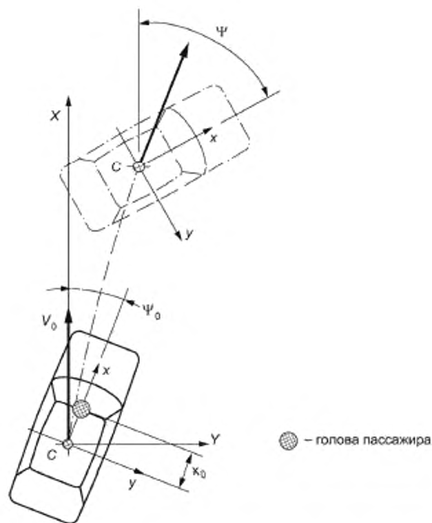
Рисунок Б.5 — Схема для расчета скорости головы в момент удара (система координат относительно транспортного средства)
