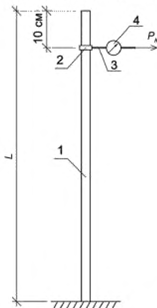
Рисунок В.1 — Схема определения нагрузки на вершину композитных опор
