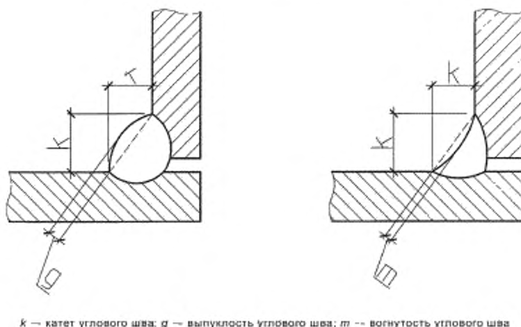
Рисунок А.1 — Схема измерения катета выпуклости и вогнутости угловых швов сварных соединений
