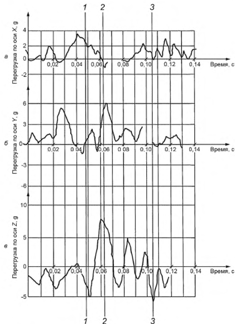
Рисунок Б.4 — Пример диаграммы ускорений (перегрузок) в центре масс по осям X (а), Y (б) и Z (в)
