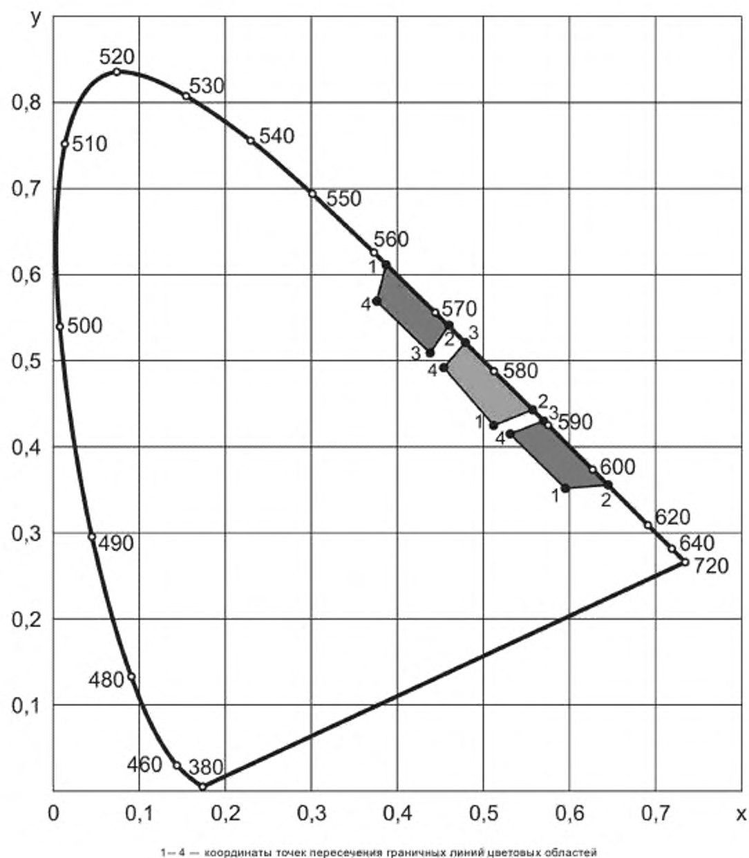
Рисунок Е.5 — График цветовой области изображений дорожных знаков (световозвращающий материал III класса со свойствами флуоресценции)
