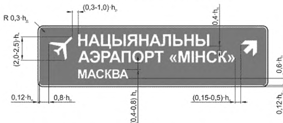
Рисунок В.2 — Пример компоновки изображения знака вида 29
