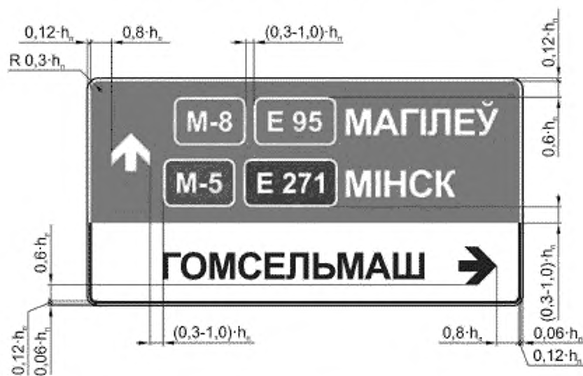
Рисунок В.4 — Пример компоновки изображения знака вида 30
