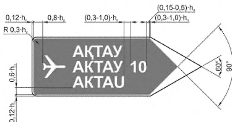
Рисунок В.3 — Пример компоновки изображения знака вида 29
