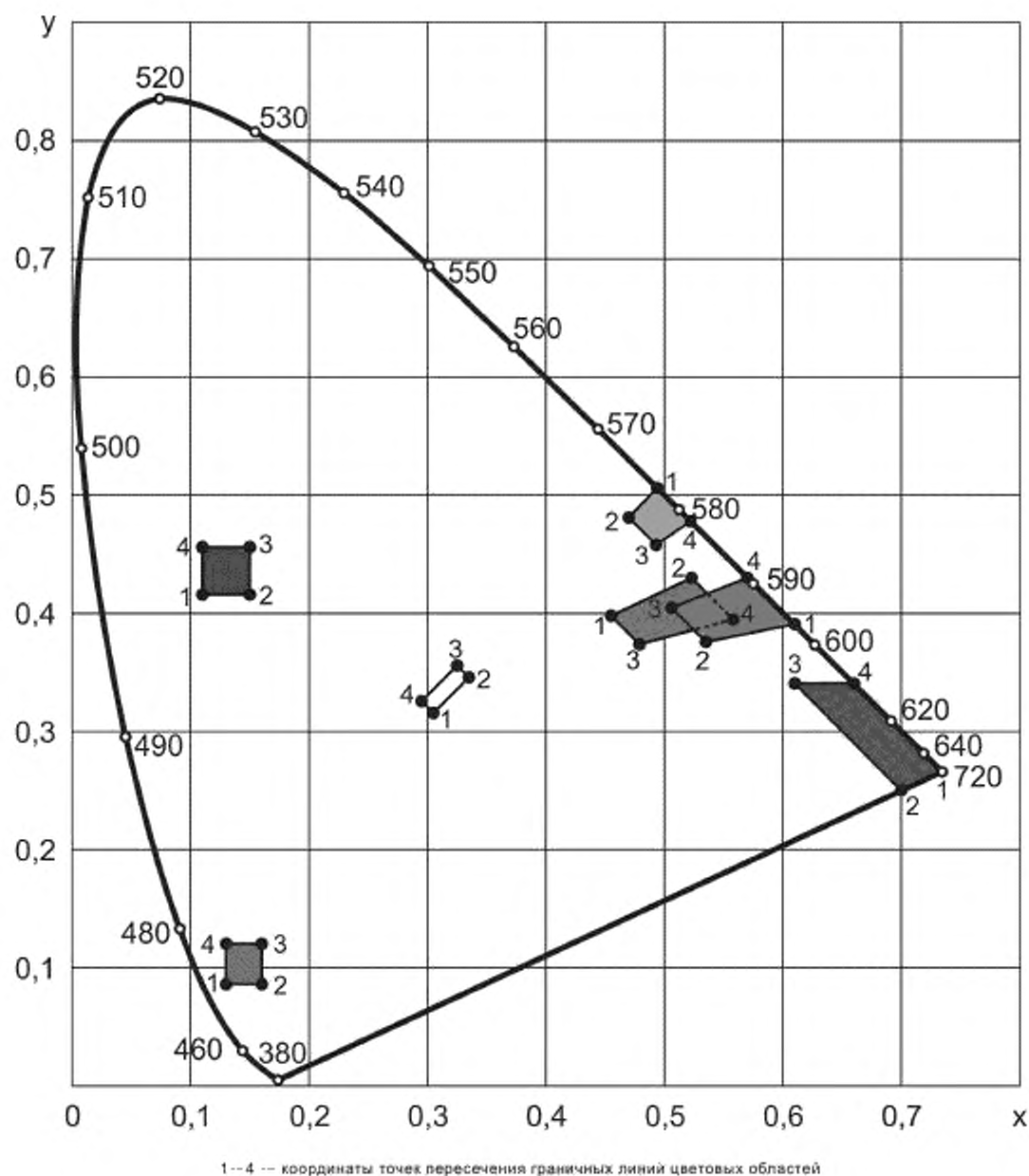
Рисунок Е.2 — График цветных областей изображений дорожных знаков (световозвращающий материал I класса с высокой цветоустойчивостью)
