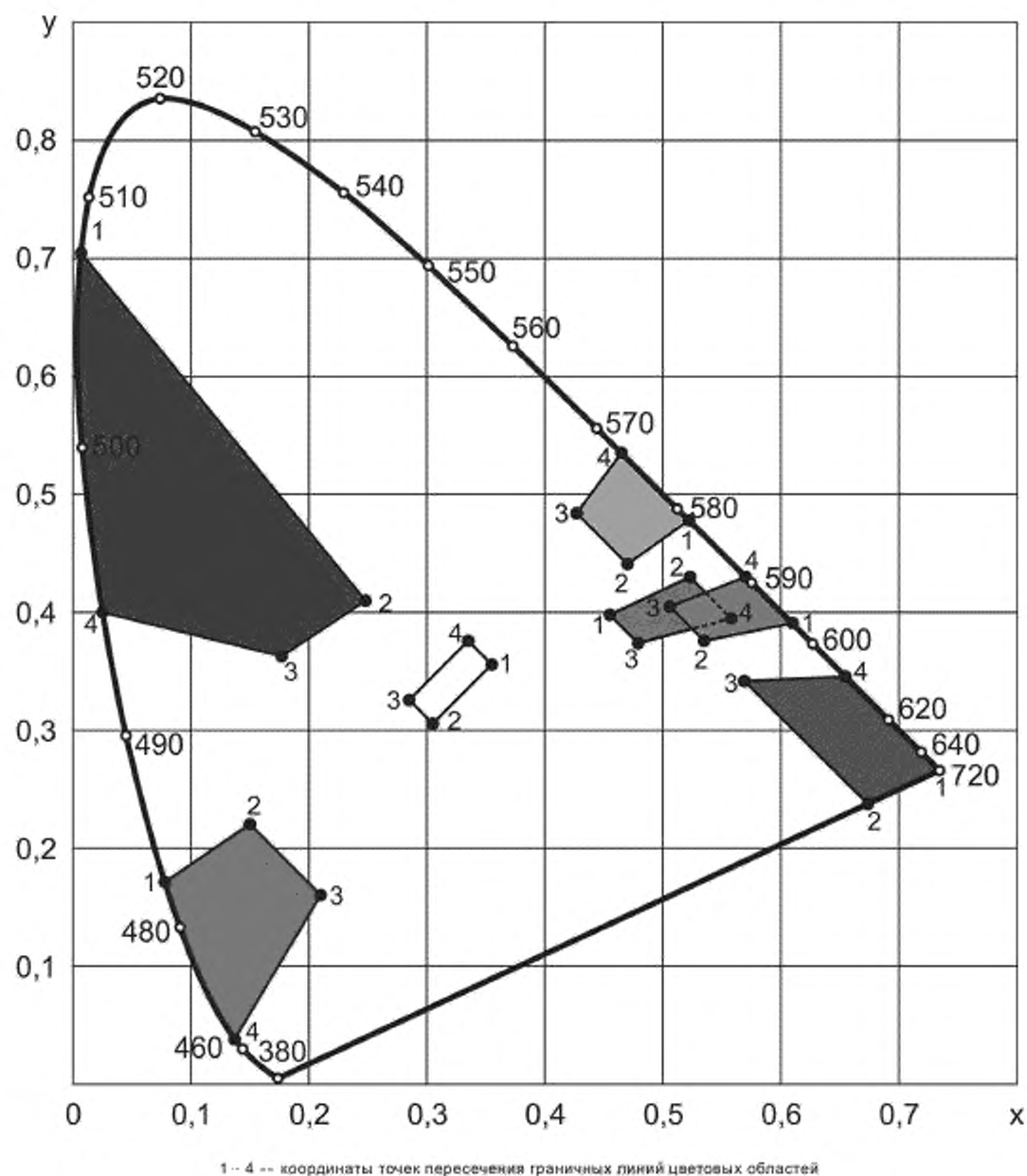
Рисунок Е.3 — График цветовой области изображений дорожных знаков (световозвращающий материал II класса со средней цветоустойчивостью)
