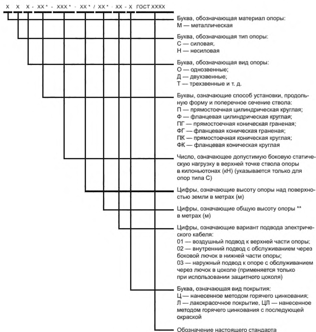
Рисунок 4.1 — Структурная схема маркировки металлических опор
