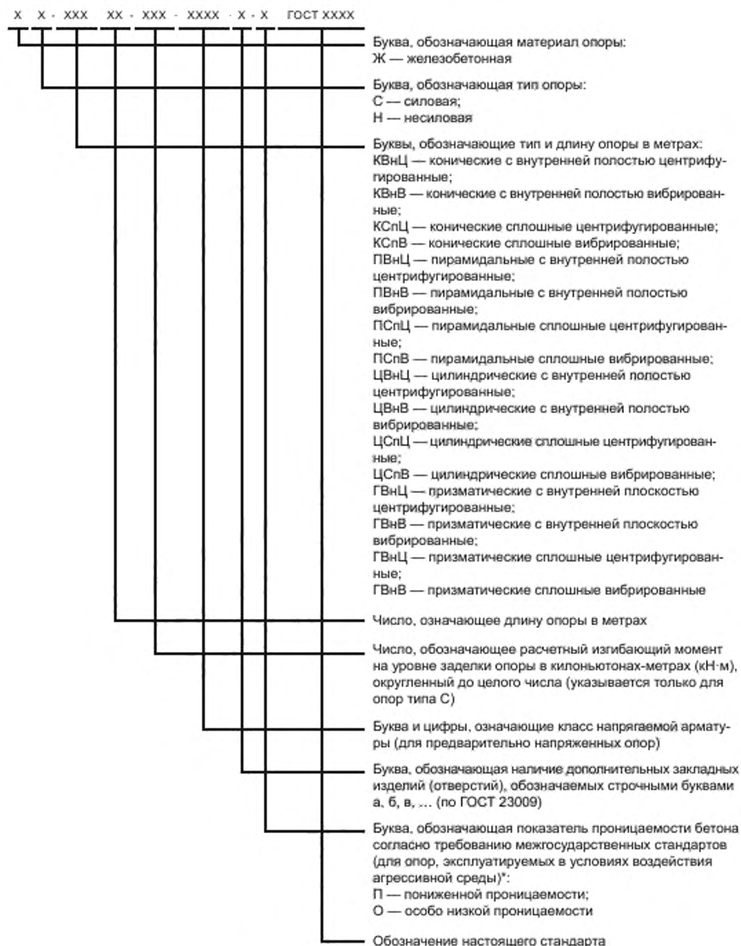
Рисунок 4.2 — Структурная схема маркировки железобетонных опор
