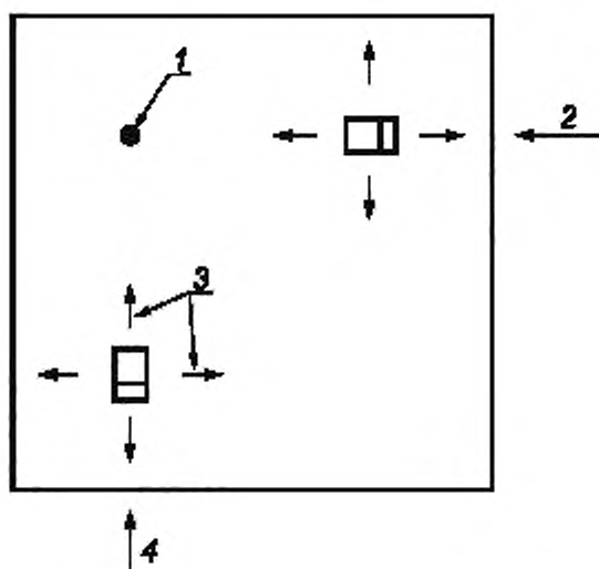
1 — несплошность; 2 — направление сканирования 1, 3 — перемещения преобразователя; 4 — направление сканирования 2
