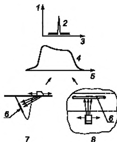
1 — амплитуда; 2 — развертка типа A; 3 — интервал; 4 — изменение максимальной амплитуды сигнала; 5 — положение преобразователя; 6 — отражатель; 7 — типичная картина в направлении по толщине; 8 — типичная картина в боковом направлении (по длине)
