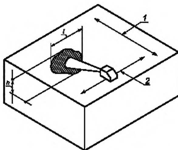
Рисунок 2 — Параметры проекции l и h для обычного определения размера несплошности с помощью наклонного преобразователя
