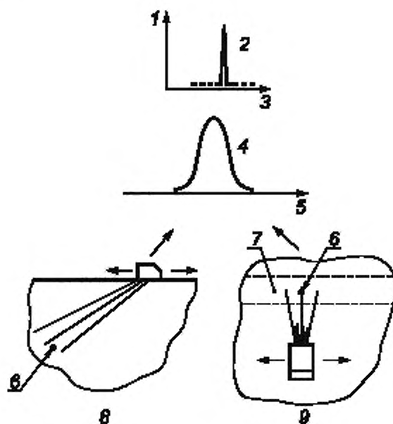
1 — амплитуда; 2 — развертка типа A; 3 — интервал; 4 — изменение максимальной амплитуды сигнала; 5 — положение преобразователя; 6 — отражатель; 7 — сварной шов; 8 — типичная картина в направлении по толщине; 9 — типичная картина в боковом направлении (по длине)
