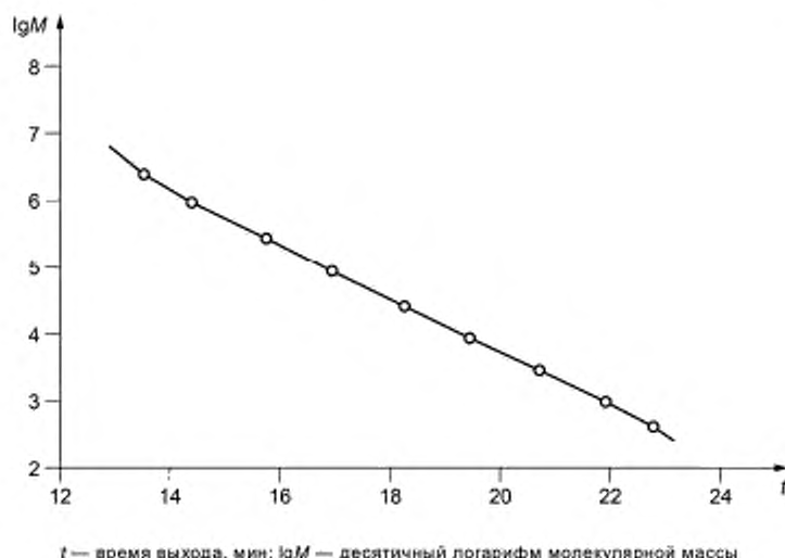
Рисунок 5 — Калибровочная кривая
