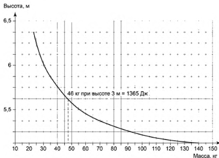
а) Нормативная кривая для энергии уровня I, требуемая энергия: 1365 Дж
