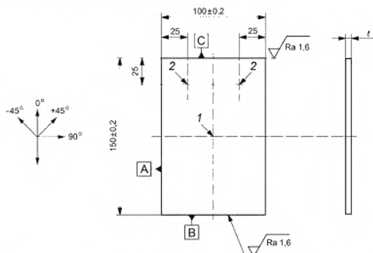
1 — точка удара, 2 — расположение тензометров; А, В, С — торцевые поверхности образца для испытаний; t — толщина образца для испытаний; R_a — шероховатость поверхности
