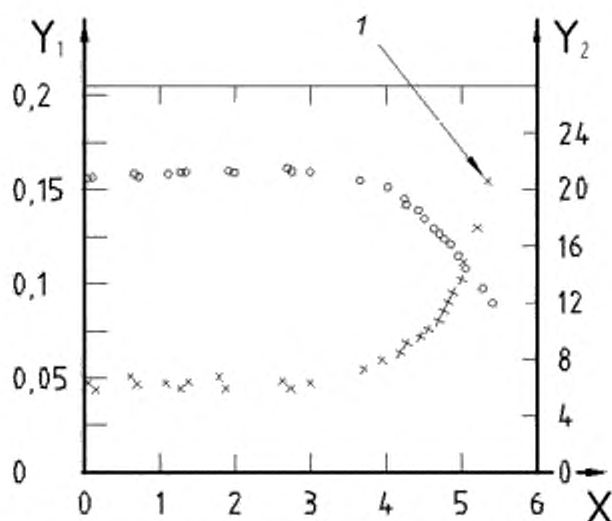
Рисунок В.2 — Динамический модуль упругости и изменения затухания
