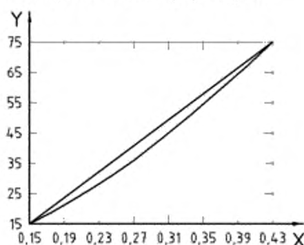
Рисунок В.1 – Типовая петля гистерезиса
