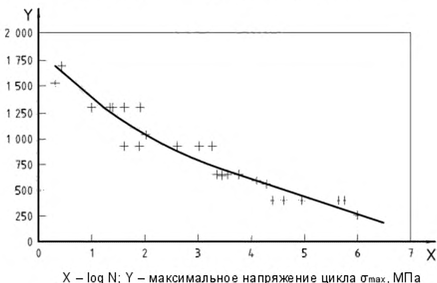
Рисунок 1 – Пример кривой усталости
