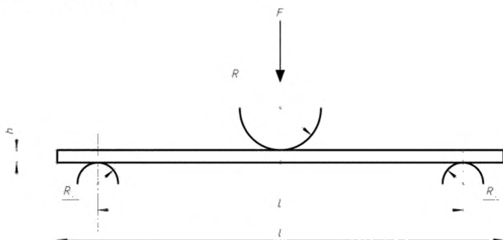
Рисунок ДА.1 – Схема трехточечного нагружения
