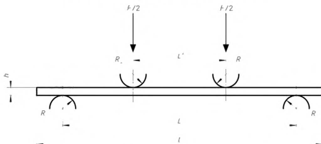
Рисунок ДА.2 – Схема четырехточечного нагружения
