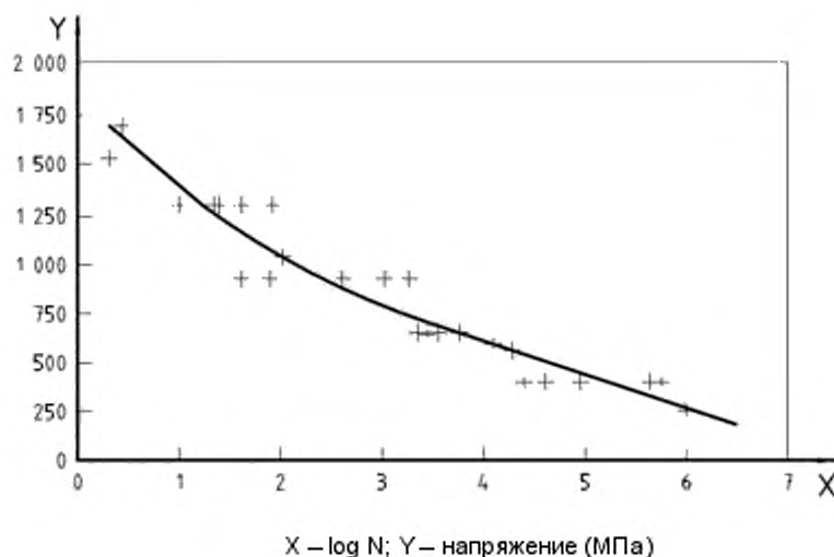
Рисунок 3 –Пример диаграммы усталости
