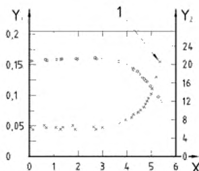
Рисунок А.2 — Динамический модуль упругости и изменение затухания
