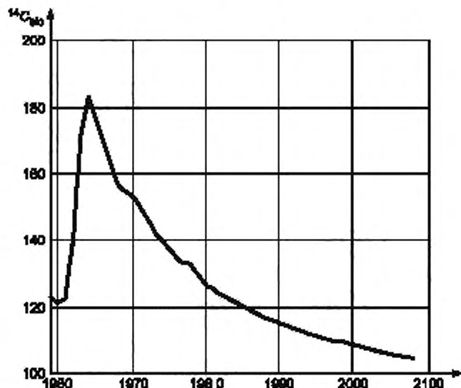
Рисунок Е.1 — Уменьшение значения ^{14}\text{C}_{\text{биоС}} в атмосферном воздухе с \text{CO}_2 (в \text{pmC} ), измеренное на высокогорной альпийской станции в Вермунте (Австрия) и Jungfraujoch (Швейцария) (см. [14], для данных 2004—2008 гг. см. сообщение С. Пэлстрой и И. Левина)
