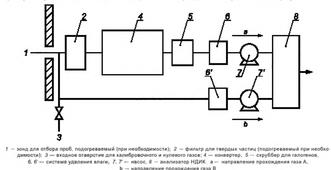
Рисунок 1 — Схема измерительной системы (пример)
