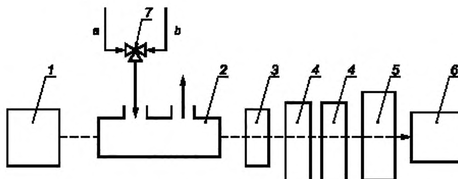
1 — источник ИК излучения; 2 — ячейка с пробой; 3 — фильтрующая ячейка или оптический фильтр; 4 — детектор; 5 — усилитель; 6 — дисплей; 7 — вентиль с плавным регулированием; а — направление газа А, b — направление газа В
