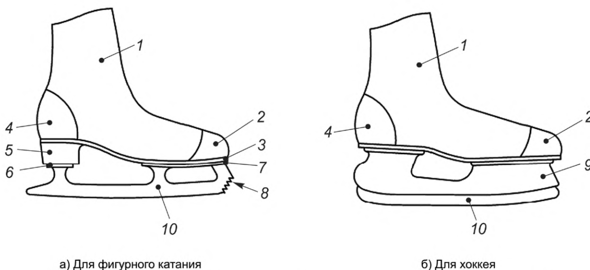
Рисунок 1 — Основные элементы несъемных коньков
