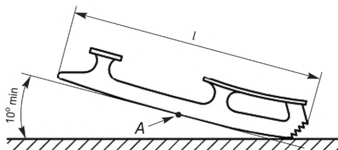
Рисунок 2 — Касание льда нижним зубом полоза конька
