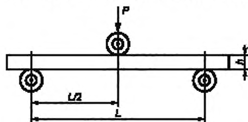
Рисунок 2 — Схема испытания образца
