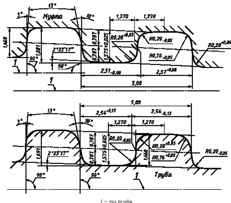
Рисунок 6 — Профиль упорной резьбы обсадных труб для размеров от 406,4 мм и более
