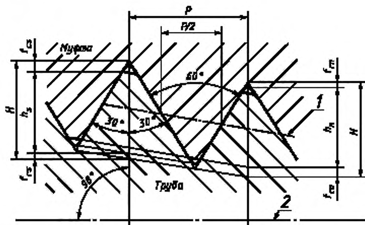
Рисунок 1 — Профиль резьбы трубопроводов
