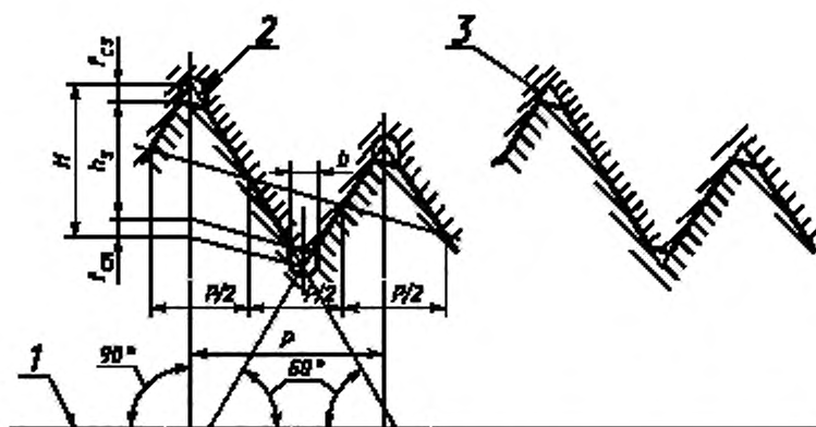
1 — ось резьбы; 2 — впадина с канавкой; 3 — заостренная впадина
