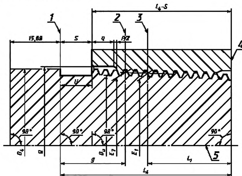
Рисунок 11 — Основные размеры калибров для контроля резьбы трубопроводов и закругленной треугольной резьбы труб
