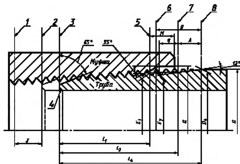
1 — плоскость середины муфты; 2 — торец трубы при механическом свинчивании; 3 — торец трубы при свинчивании от руки; 4 — внутренняя фаска у торца трубы; 5 — плоскость свинчивания от руки; 6 — основная плоскость; 7 — плоскость начала сбега резьбы; 8 — плоскость конца сбега резьбы
