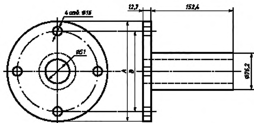
Рисунок 15 — Поддерживающий фланец для калибров
